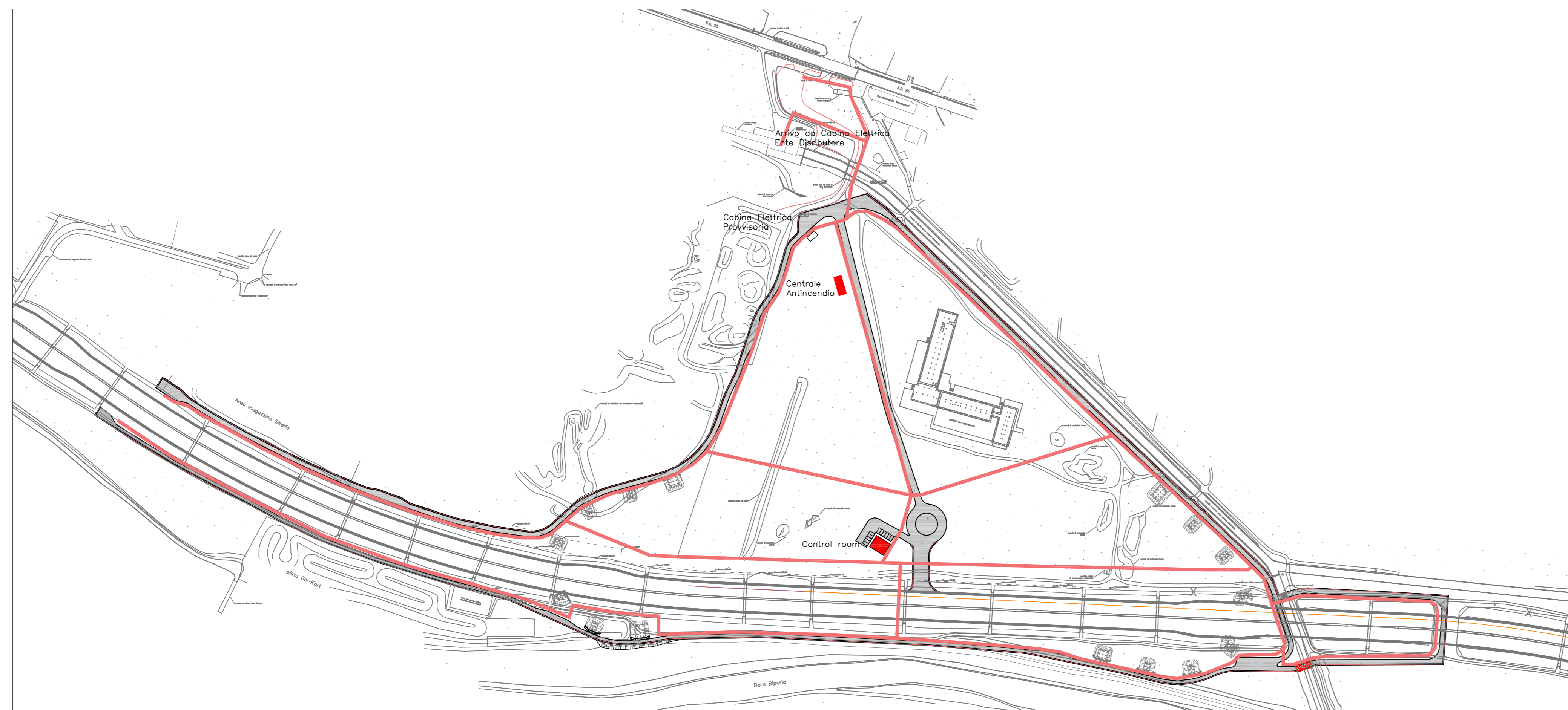
COPERTURA VIDEOSORVEGLIANZA TELECAMERE PTZ DOME PERIMETRALI
