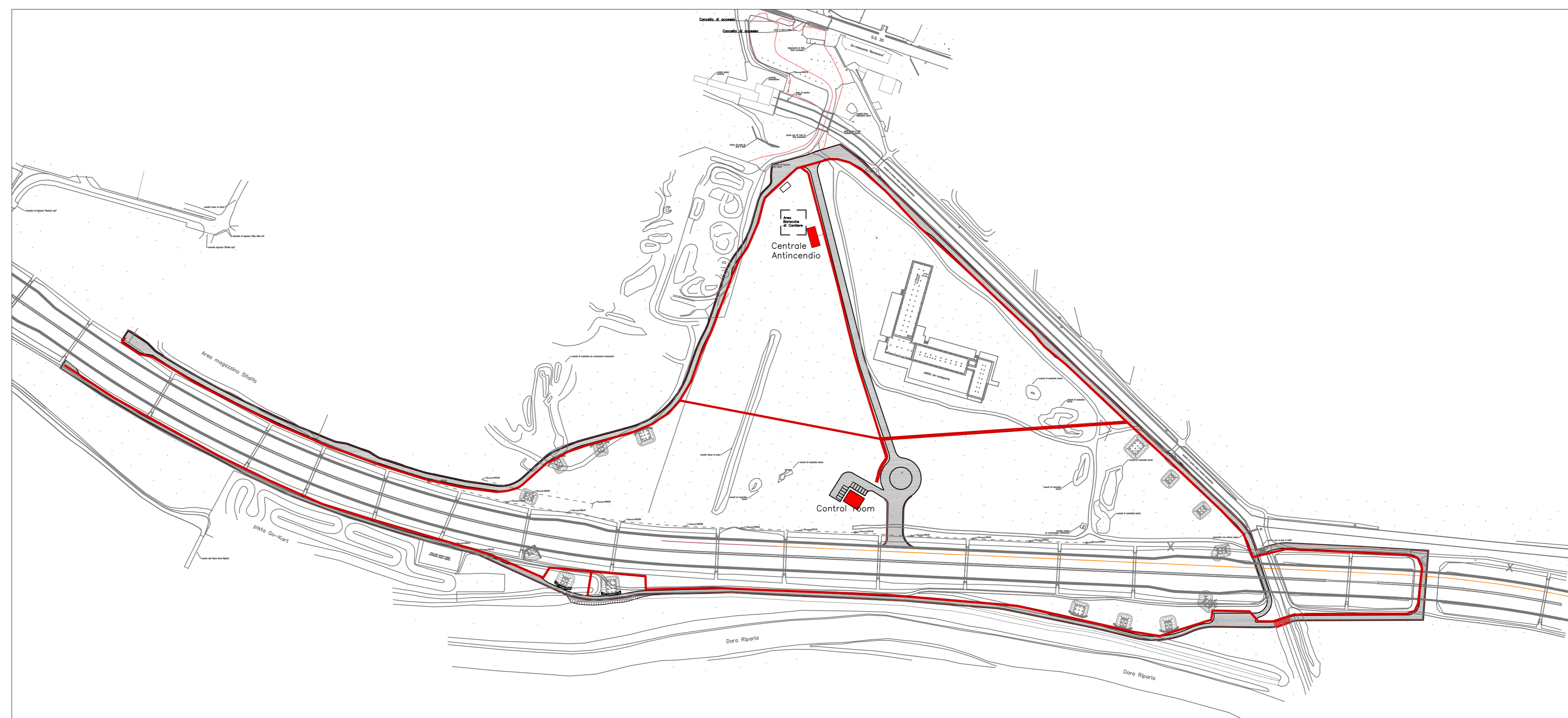
COPERTURA RETE IDRANTI PERIMETRALI
