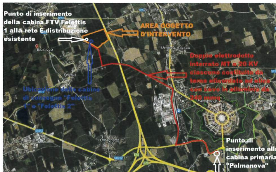
Figura 2 Vista di insieme dell’impianto di connessione con collegamento cavi MT interrati (in rosso) su base ortofoto (Cfr. Relazione paesaggistica) Di seguito viene rappresentata l’intera planimetria di intervento in cui sono rappresentati, oltre che la zona, anche i percorsi delle linee elettriche interrate e la zona di connessione alla rete elettrica nazionale.
