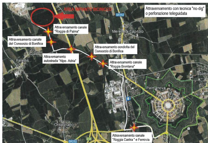
Figura 5 Interferenze del cavidotto con la rete idraulica e le infrastrutture del territorio del territorio
