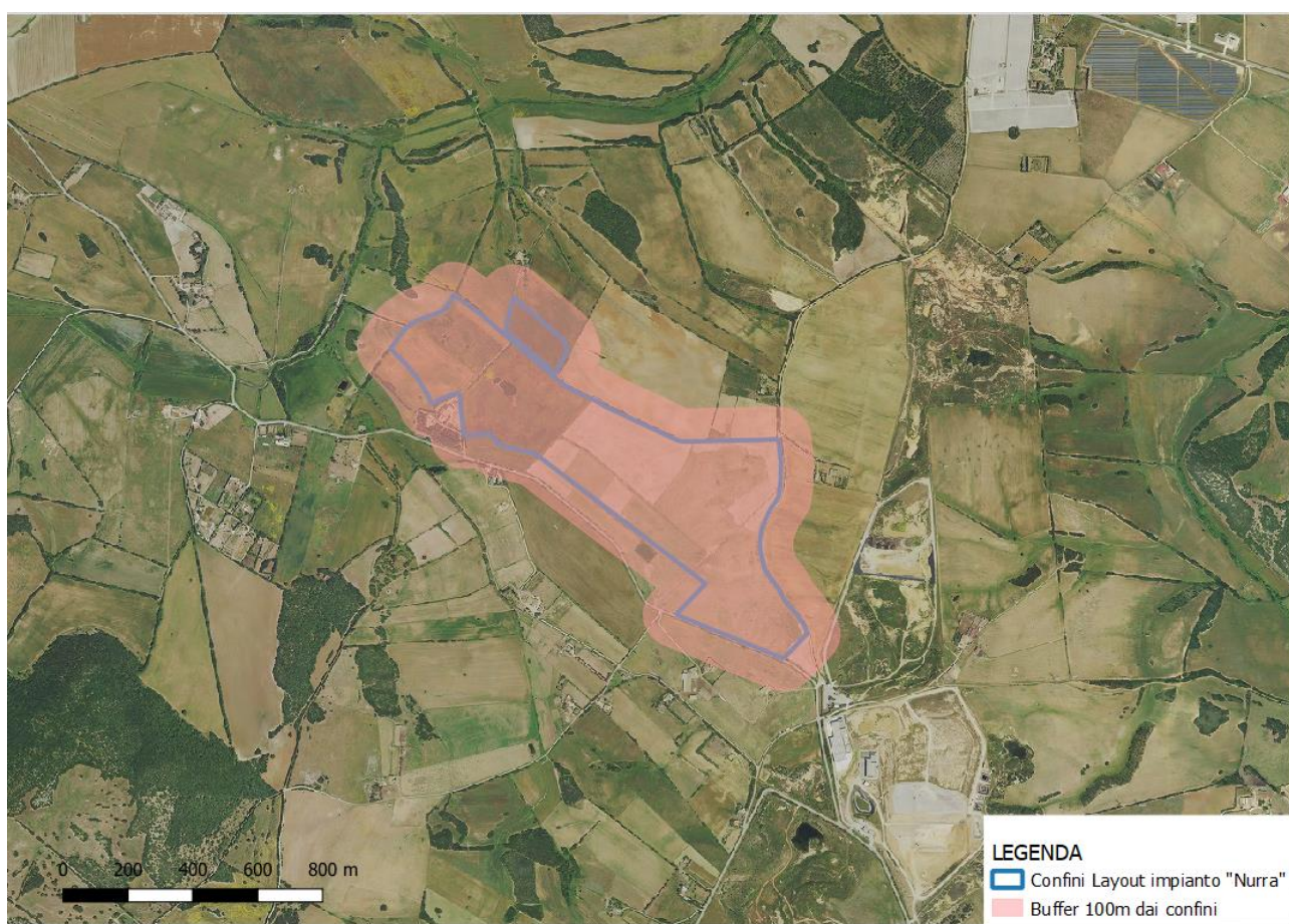
Figura 4 – Ambito di interazione con il paesaggio agricolo individuato entro un areale di 100 metri dall'impianto agrivoltaico in progetto
