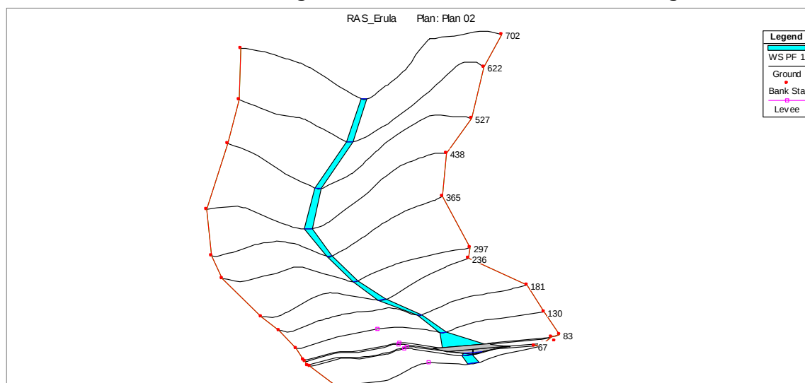
Rappresentazione 3D – River 1 (Bacino 1)
