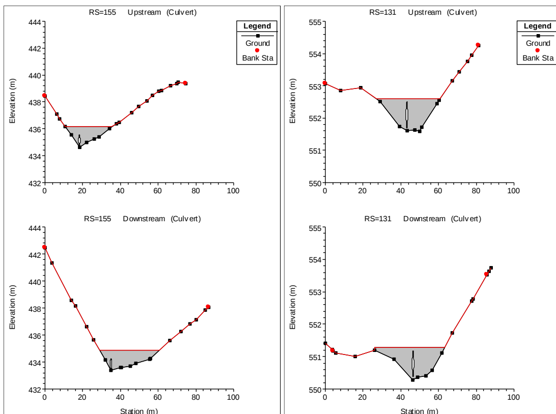
Attraversamenti River 4 (a sinistra) e River 5 (a destra).
