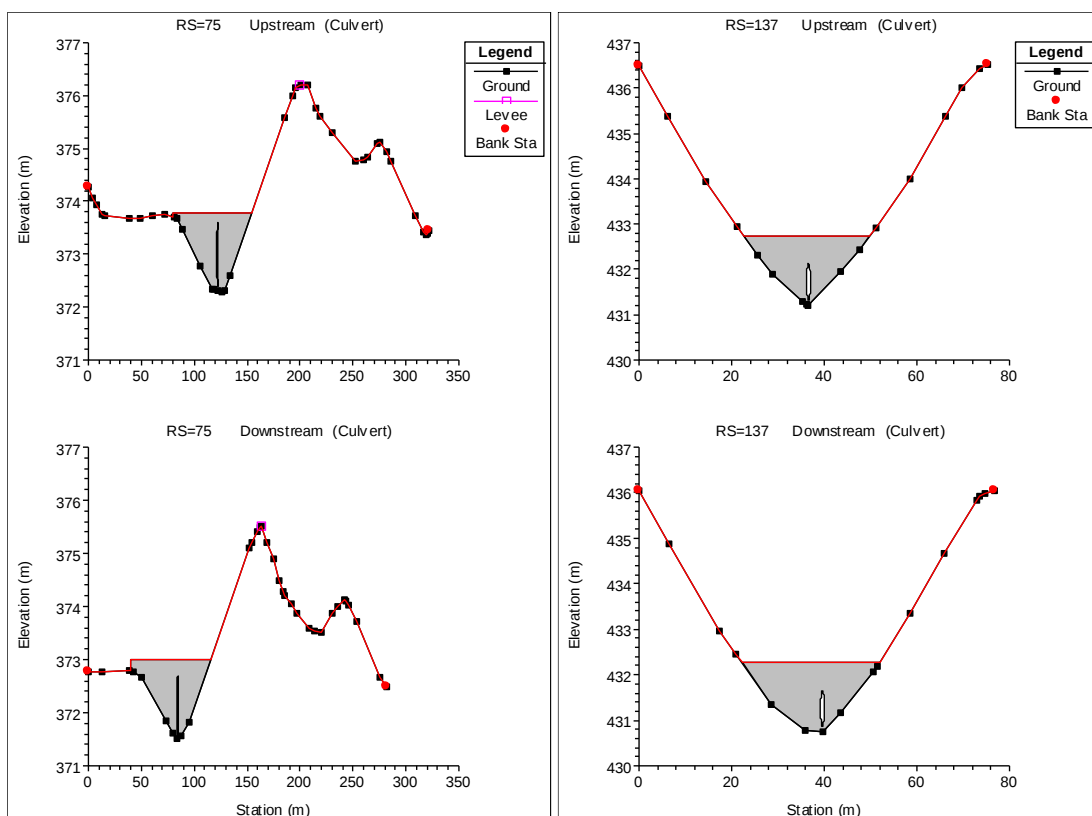
Attraversamenti River 1 (a sinistra) e River 2 – Lower (a destra).
