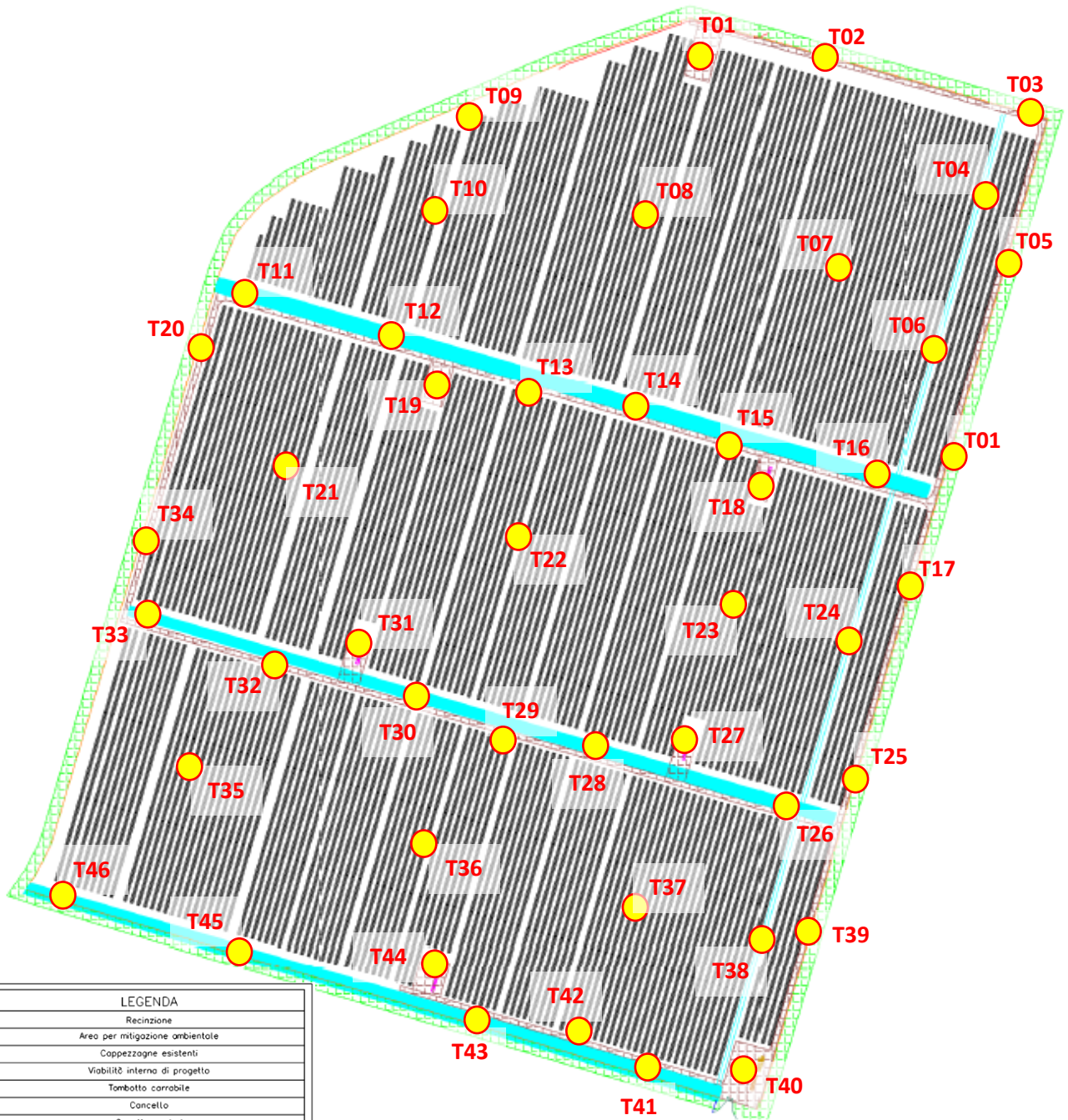
Figura 7 - Idraulica Bondeno Nord
