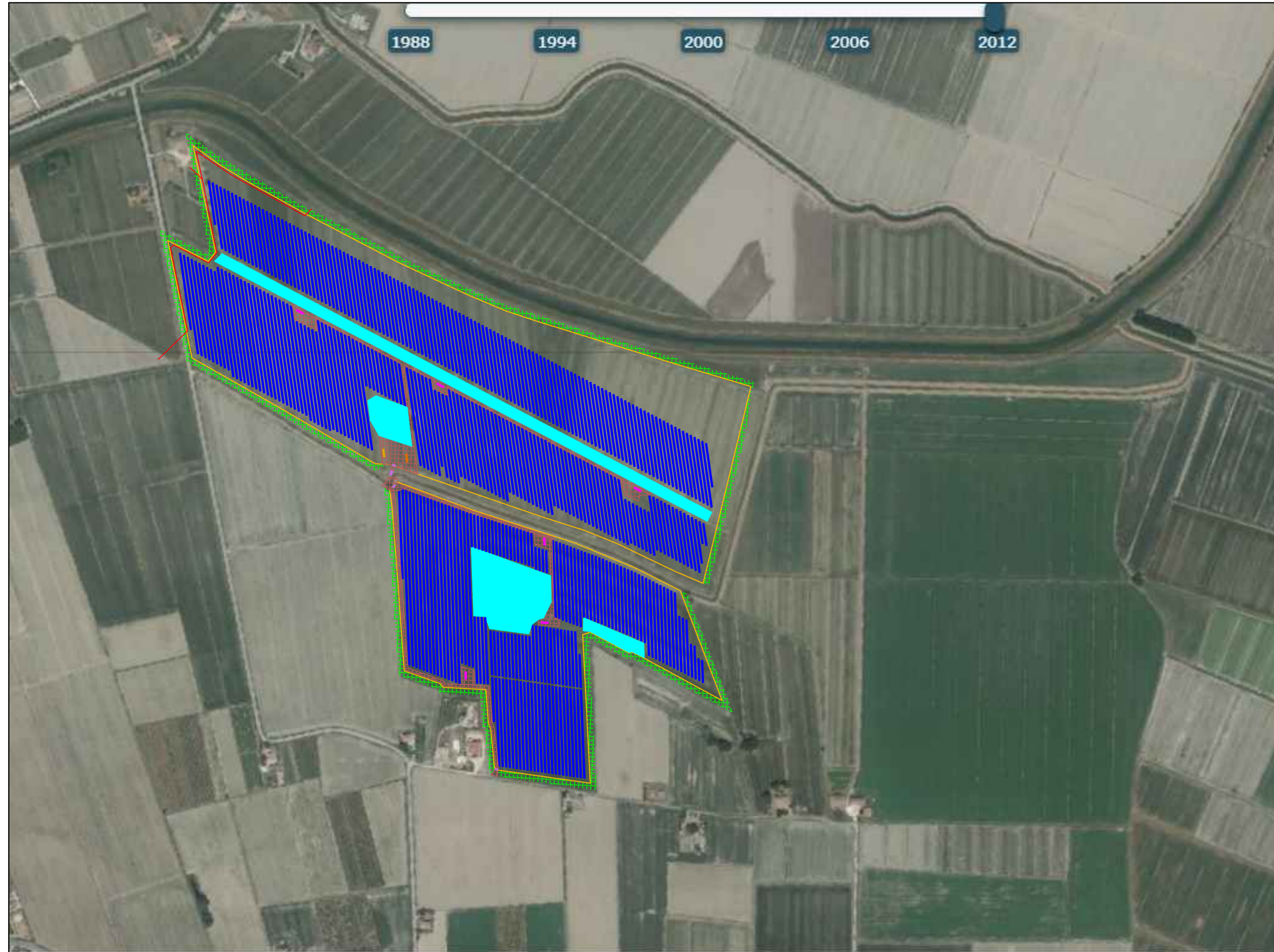
Impianto sud - Stato di progetto
