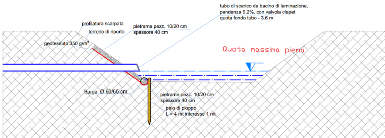
Figura 5.1 - Sezione tipologica punto scarico con valvola clapet e protezione spondale
