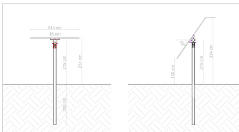
Figura 3.1-1 - Tracker tipo ad asse variabile
