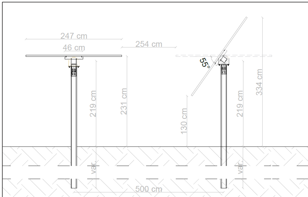
FIGURA 1: TRACKER SOLARE TIPO
