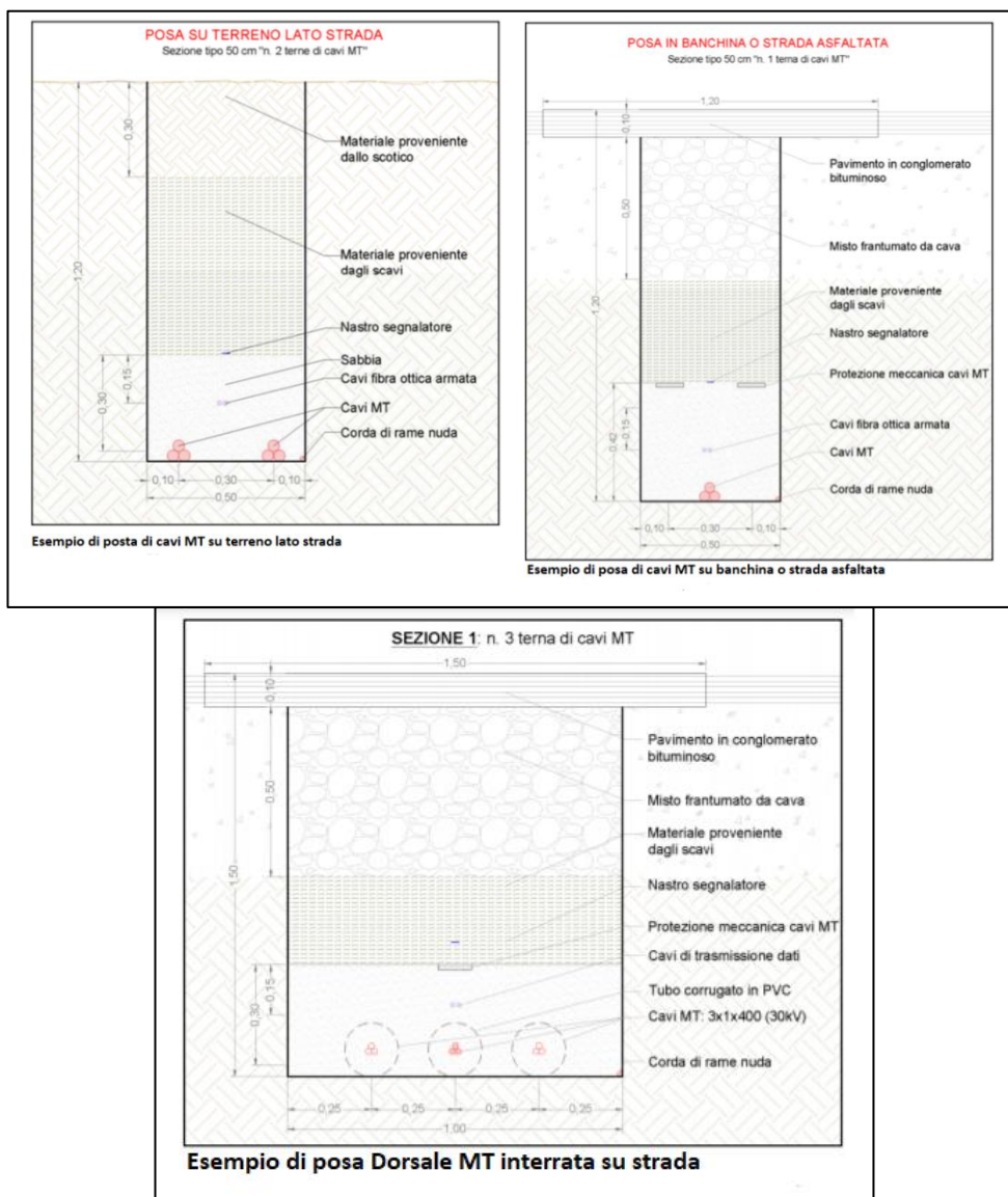
FIGURA 12: ESEMPI POSA CAVI
