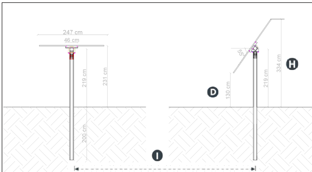
FIGURA 4: DEFINIZIONE DELLE DIMENSIONI DEI TRACKER
