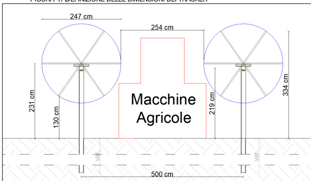
FIGURA 3: CONFIGURAZIONE STRUTTURE AD INSEGUIMENTO IMPIANTO AGRIVOLTAICO
