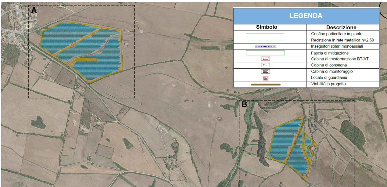
FIGURA 1 – LAYOUT PLANIMETRICO DELL'AREA D'IMPIANTO
