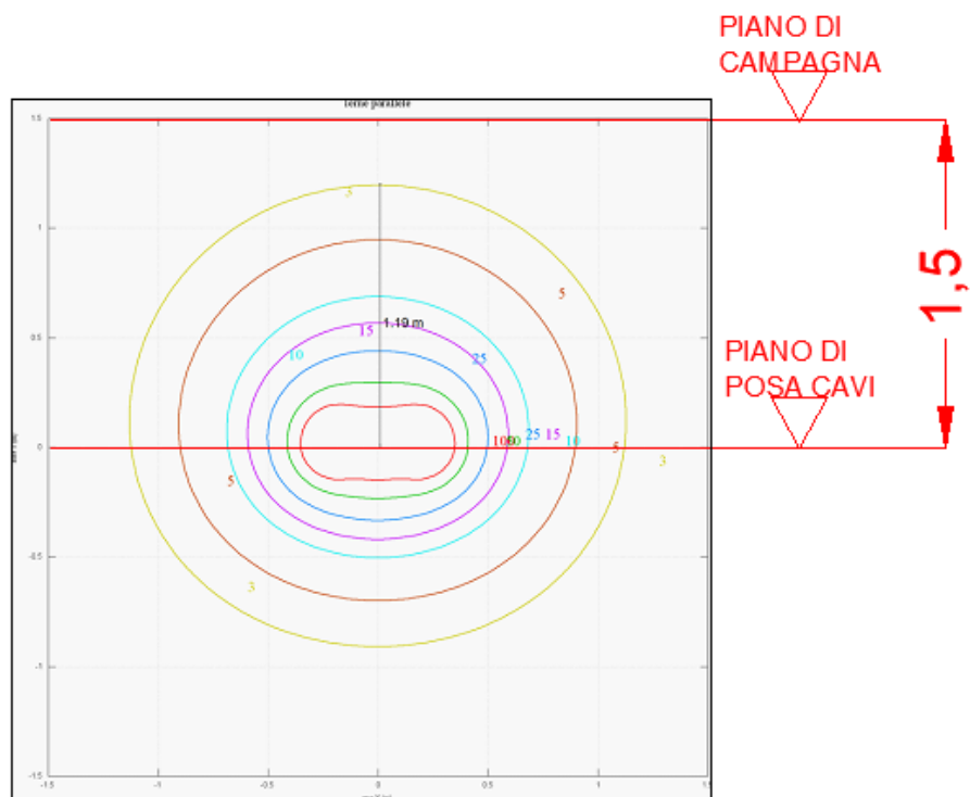
FIGURA 3: CURVE ISOINDUZIONE – 3 LINEE AT INTERRATE COLLEGAMENTO SE TERNA
