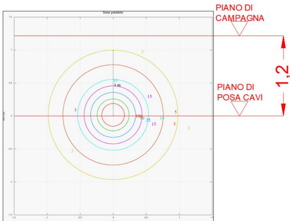
FIGURA 2: CURVE ISOINDUZIONE – 1 LINEA AT INTERRATA COLLEGAMENTO TRA CABINA DI TRASFORMAZIONE E CABINA DI CONSEGNA
