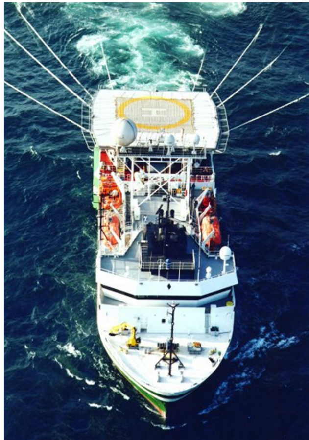
Figura 3-8: esempio di nave per ricerca geofisica impegnata in un rilievo sismico 3D con una configurazione a otto cavi (Fonte: eni s.p.a. divisione e&p)
