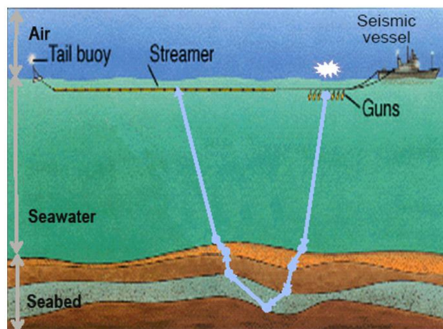
Figura 3-6: schema generale del metodo di acquisizione sismica con “air gun” e “streamer” (Fonte: eni s.p.a. divisione e&p)
