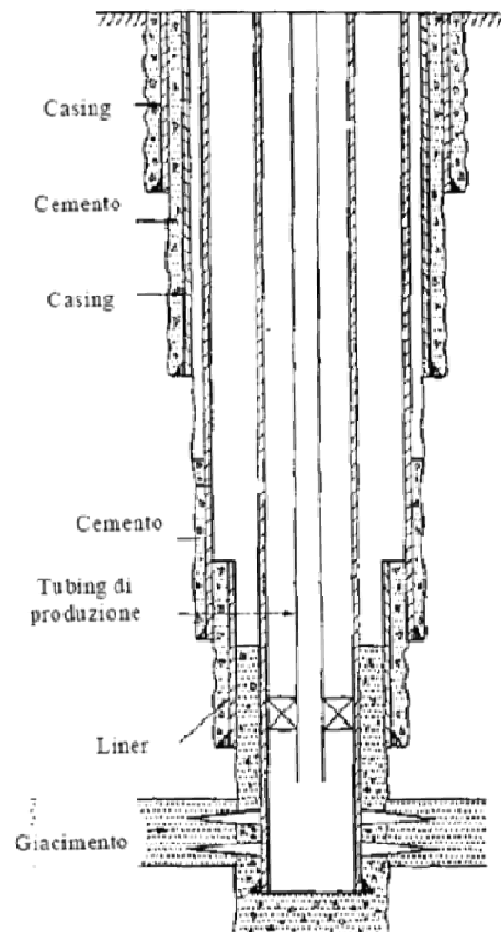
Figura 3-20: casing e cementazioni
