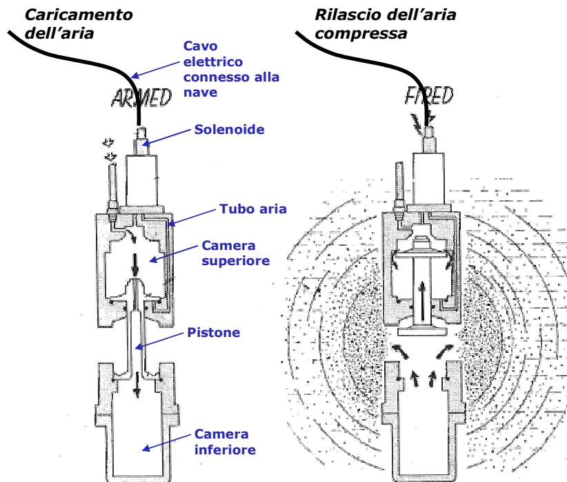
Figura 3-10: caratteristiche costruttive e funzionali di un "air gun" (Fonte: eni s.p.a. divisione e&p)
