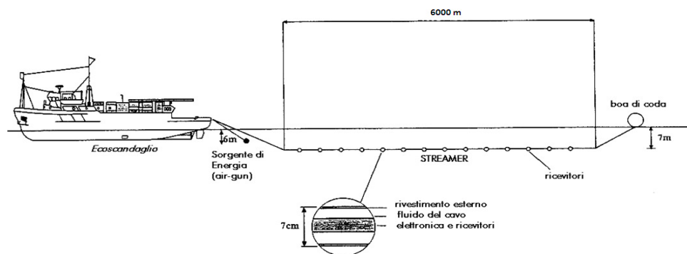
Figura 3-13: allestimento della nave sismica (Fonte: eni s.p.a. divisione e&p)
