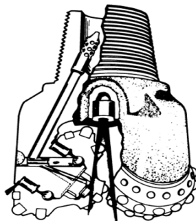
Figura 3-19: scalpello di perforazione
