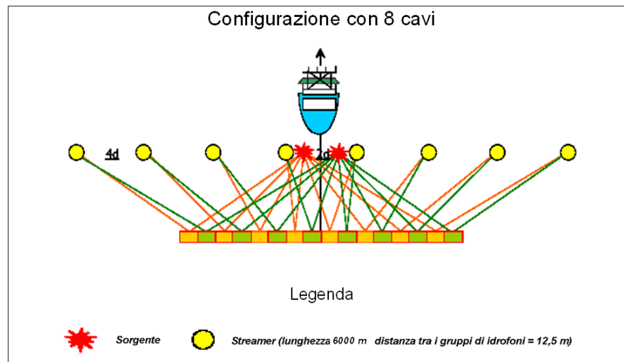
Figura 3-14: configurazione con 8 cavi prevista per l'esecuzione dei rilievi (Fonte: eni s.p.a. divisione e&p)
