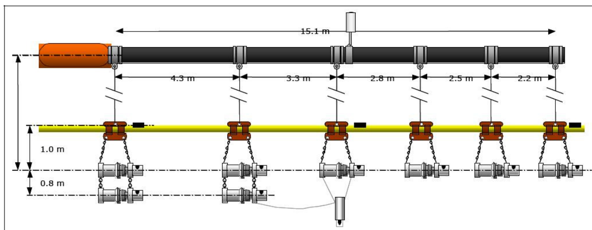
Figura 3-11: esempio di configurazione di una sorgente multipla di "air gun" (Fonte: eni s.p.a. divisione e&p)
