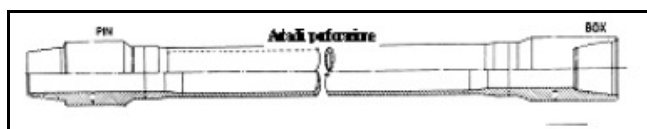
Figura 3-17: asta di perforazione
