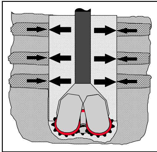
Figura 3-18: fango di perforazione in equilibrio idrostatico con i fluidi presenti negli strati rocciosi
