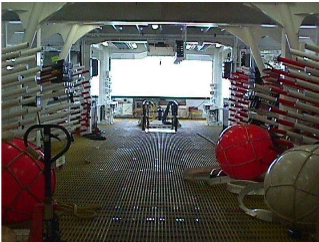
Figura 3-12: poppa di una nave per ricerca geofisica con gli stabilizzatori di profondità e le boe (Fonte: eni s.p.a. divisione e&p)
