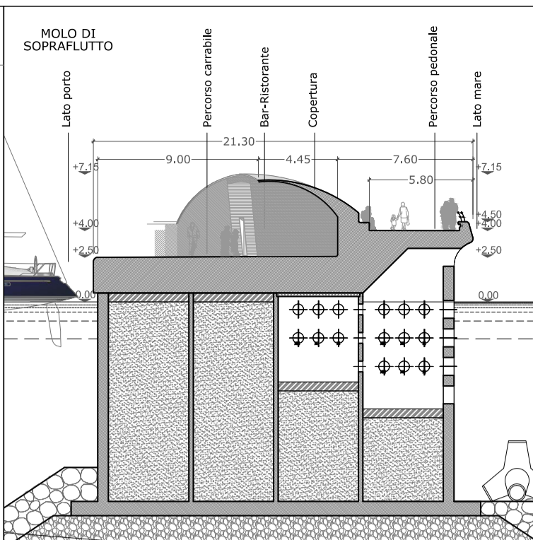
SEZIONE B - B' SCALA 1/300
