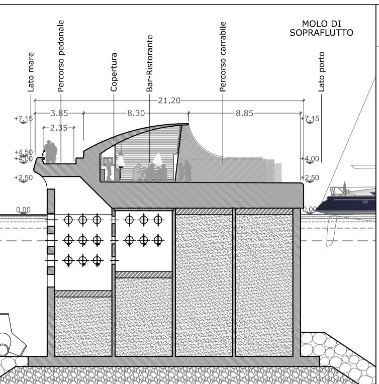
SEZIONE A - A' SCALA 1/300
