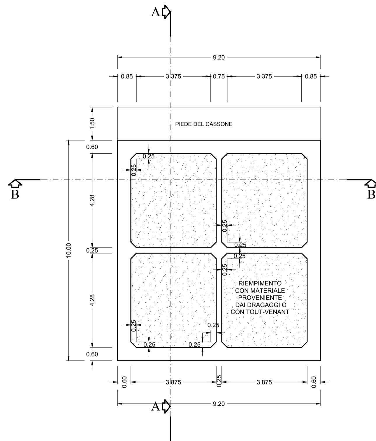
PIANTA A QUOTA -2.00 m Scala 1:100
