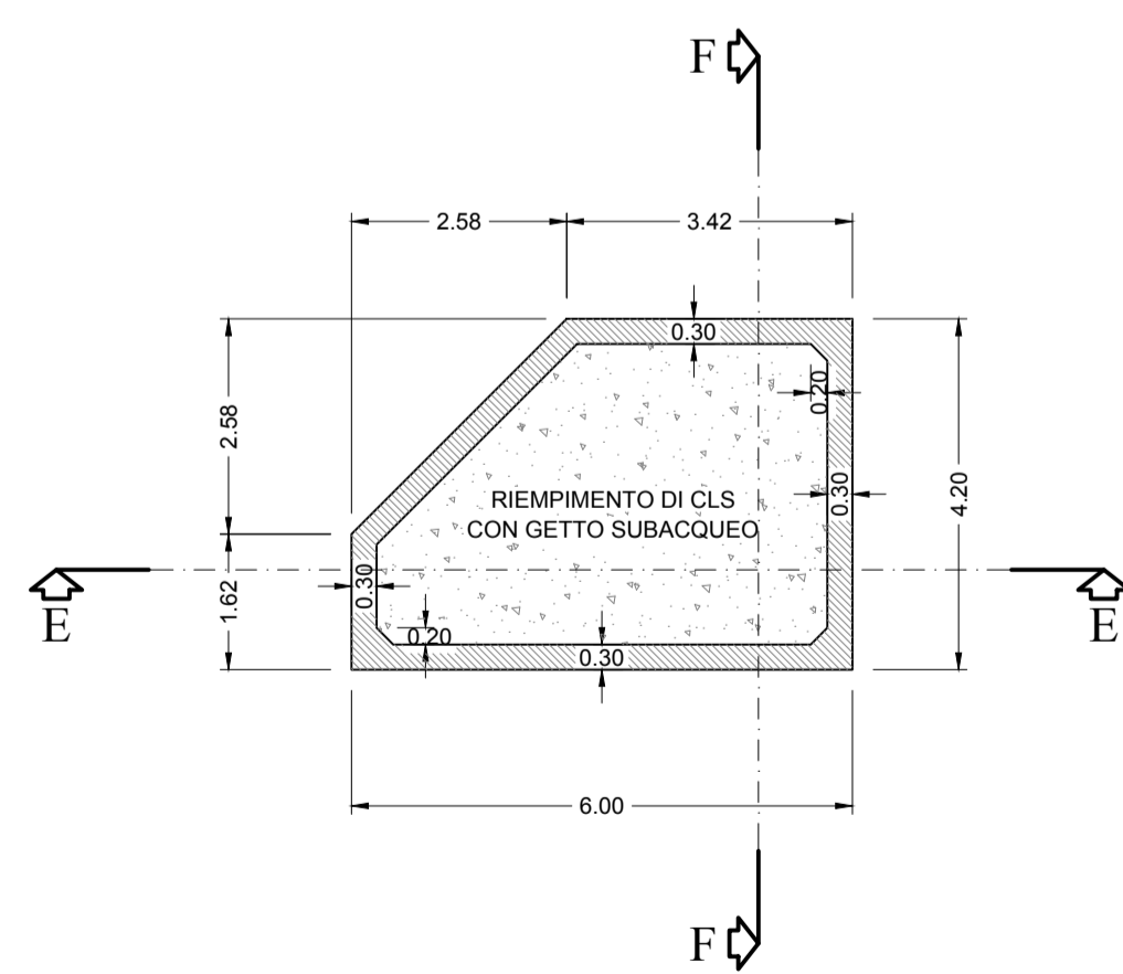
PIANTA Scala 1:100
