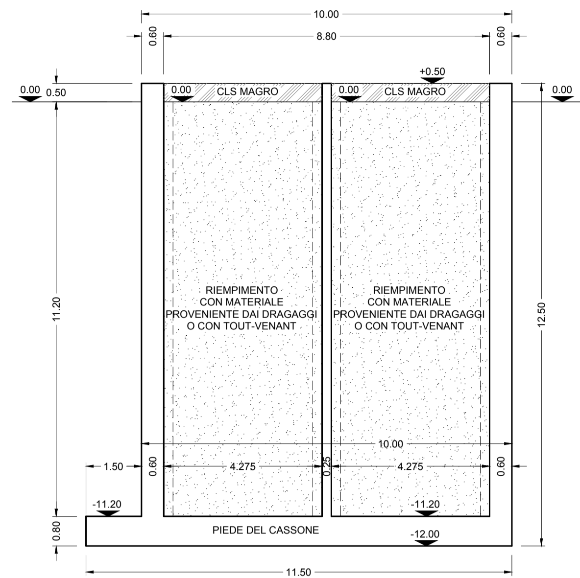
SEZIONE A - A Scala 1:100
