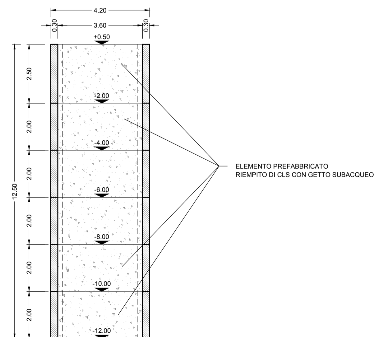
SEZIONE F - F Scala 1:100
