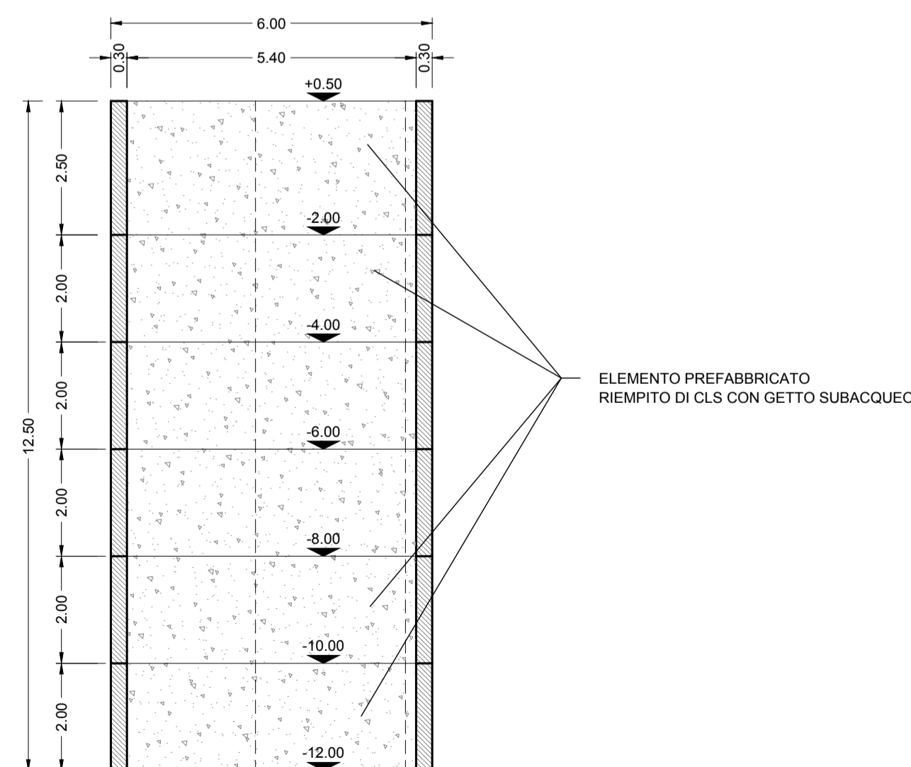
SEZIONE E - E Scala 1:100
