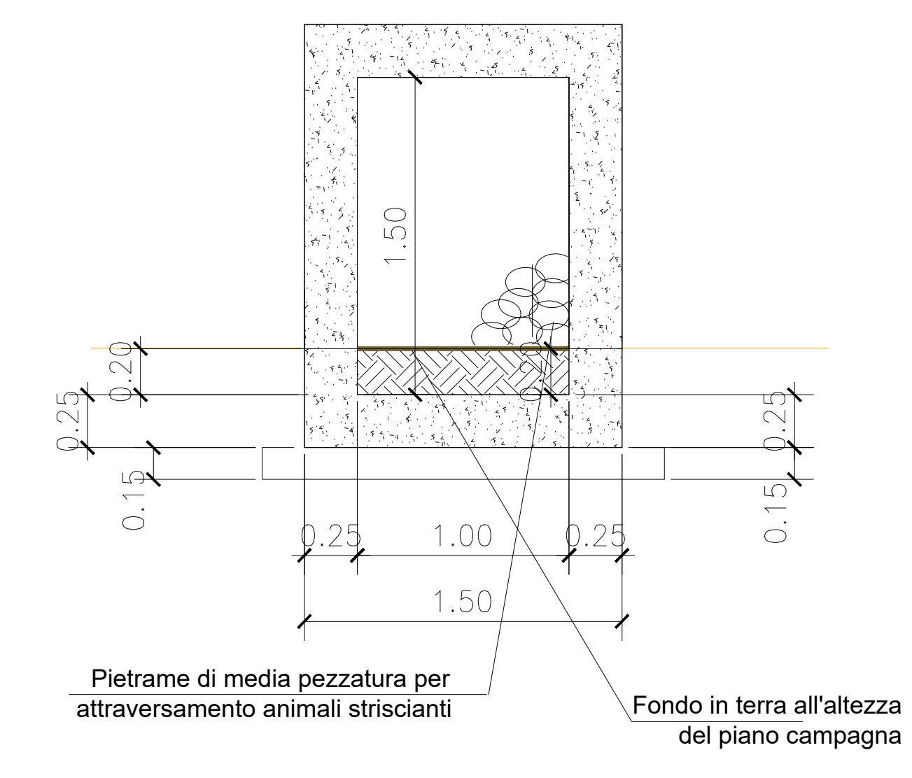
Pietrame di media pezzatura per attraversamento animali striscianti Fondo in terra all'altezza del piano campagna
