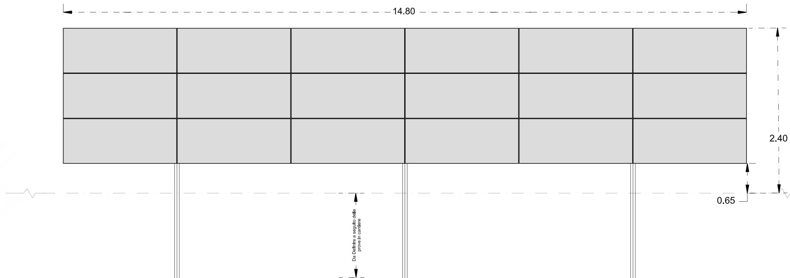
Prospetto Frontale
