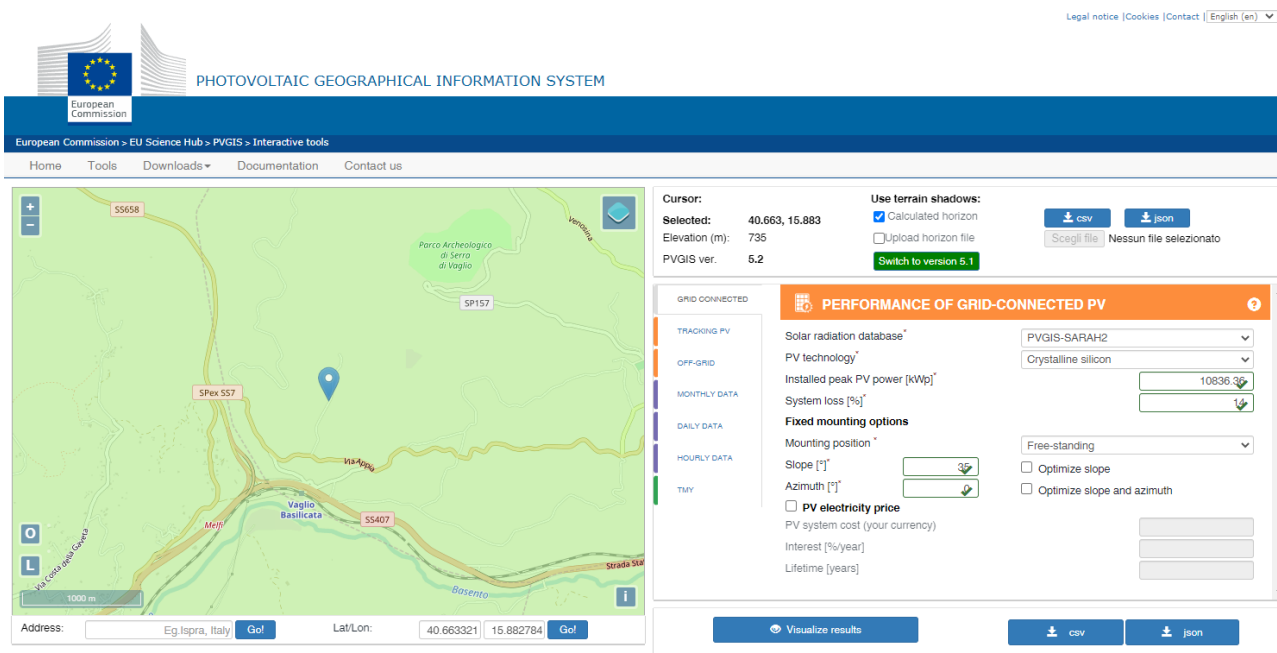
Figura 3.3b. – Inserimento nell’applicativo della localizzazione dell’impianto e delle caratteristiche tecnico-produttive con moduli fissi nella configurazione mista.
