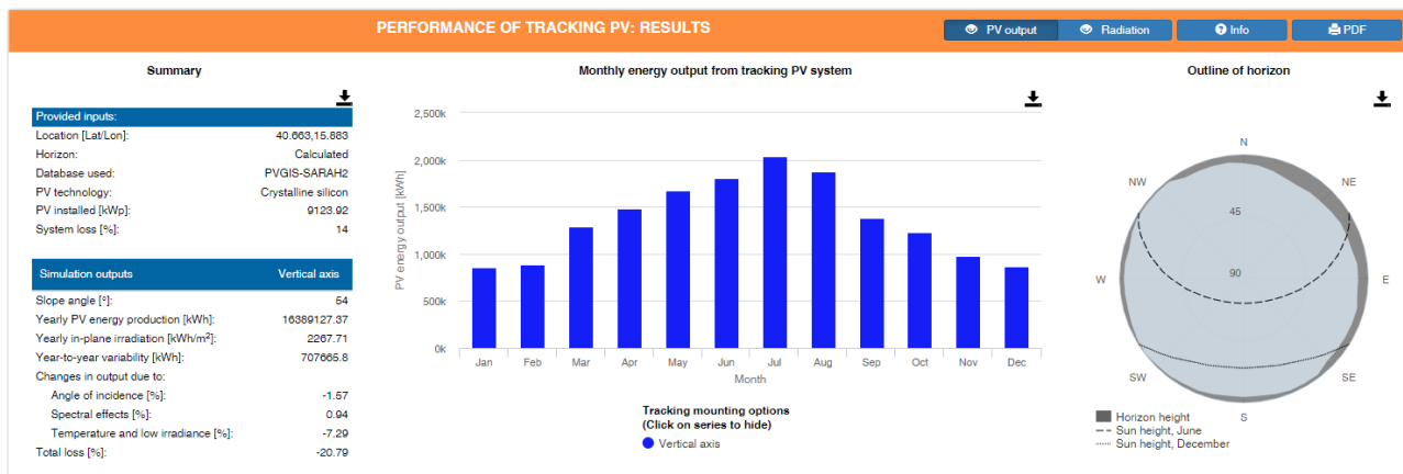
Figura 3.4a. – Rendimento dell’impianto e delle caratteristiche tecnico-produttive con tracker nella configurazione mista.
