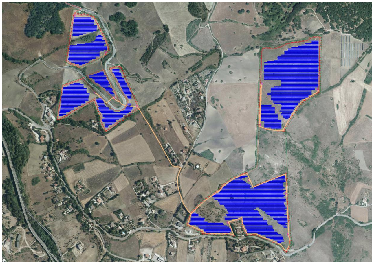
Figura 3.5. – Layout del sistema fotovoltaico con supporti fissi (area ovest).
