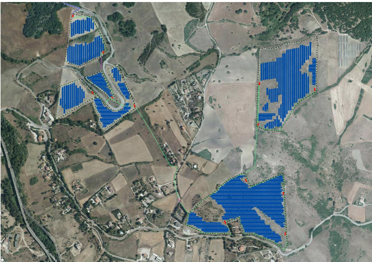
Figura 3.2. – Layout del sistema agrivoltaico con tracker e supporti fissi (mista).
