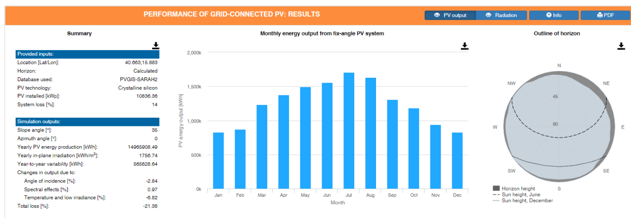
Figura 3.4b. – Rendimento dell’impianto e delle caratteristiche tecnico-produttive con moduli fissi nella configurazione mista.
