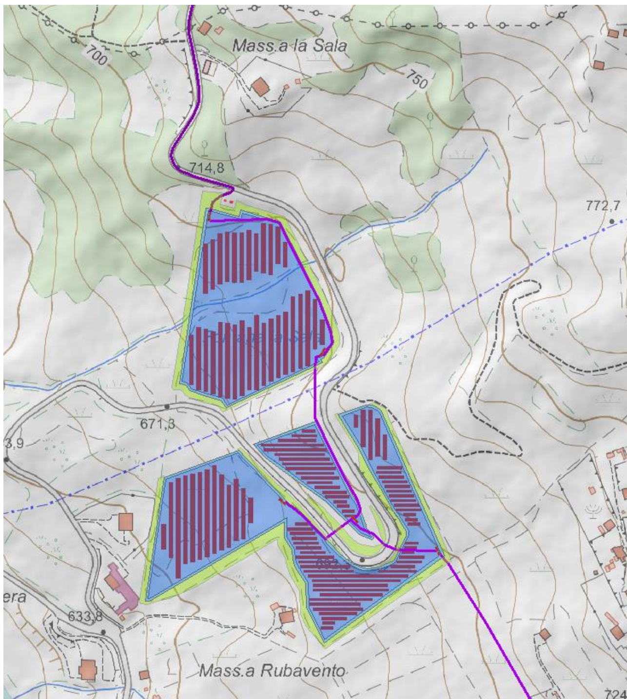
Figura 1.3a. – Individuazione dell’impianto agro-voltaico su CTR – dettaglio.
