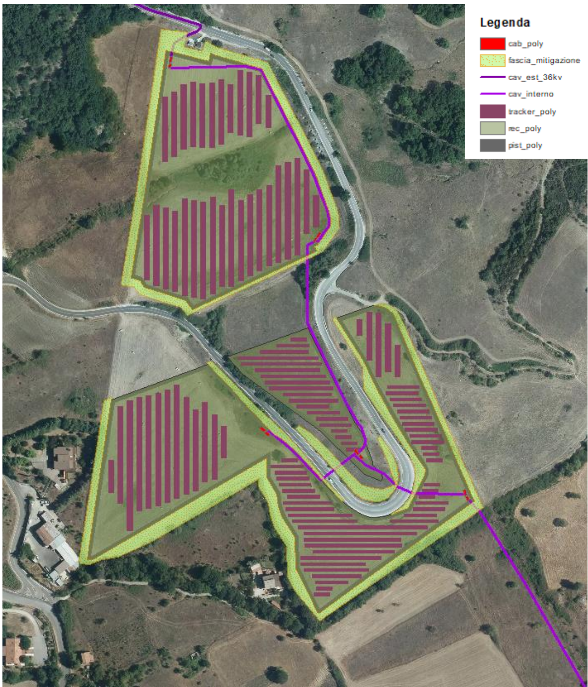
Figura 2.10. – Area di interesse dell’Impianto Agrovoltaico – dettaglio.
