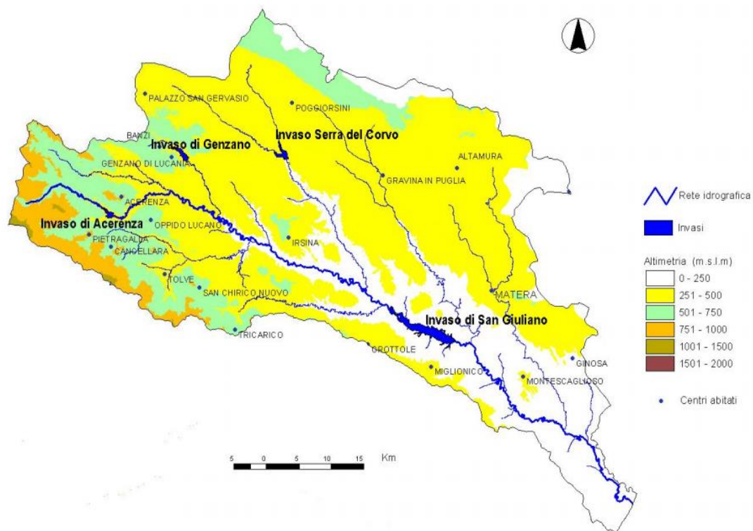
Figura 1.11. – Bacino Idrografico del fiume Bradano.
