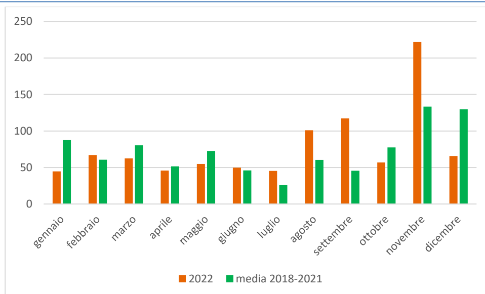
Figura 1.8 – ripartizione delle piogge nell’area Sub Appennino e Alta Valle dell’Agri -confronto anno 2022 e media del periodo 2018-2021.
