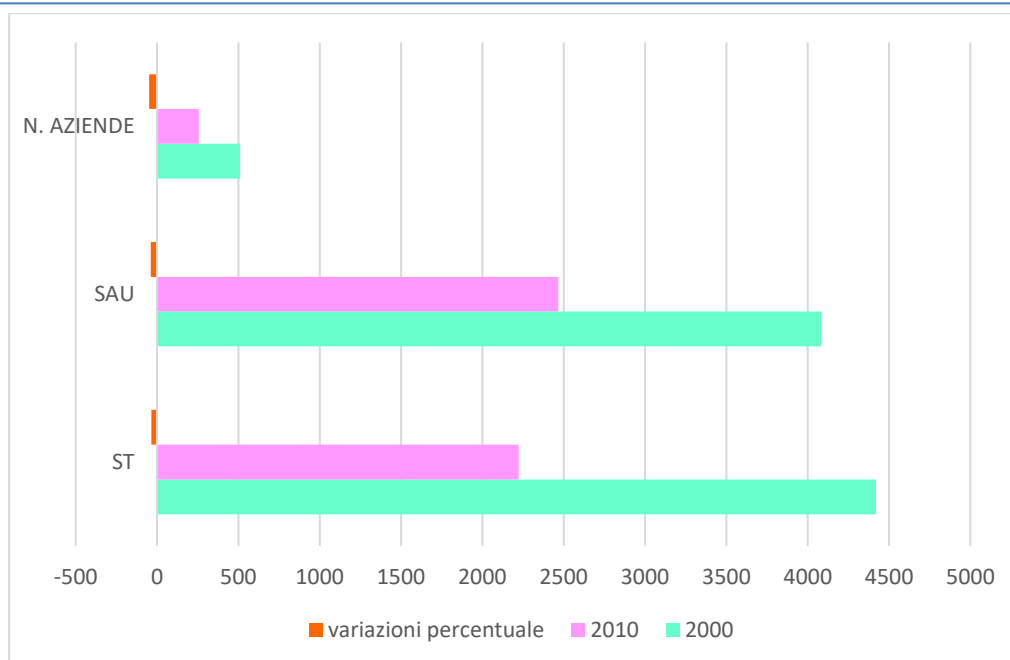
Figura 1.14. – Variazione (in valore assoluto e in percentuale) del numero di Aziende, della Superficie totale (SAT) e della Superficie agricola utilizzata (SAU) per comune: confronto censimenti 2000 -2010.
