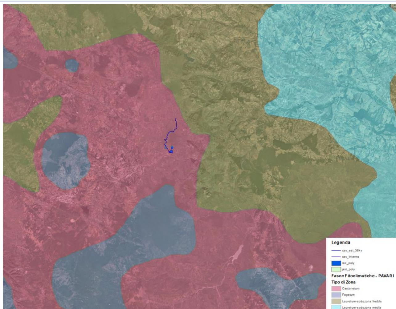
Figura 1.9. – Stralcio Carta delle fasce fitoclimatiche del Pavari.
