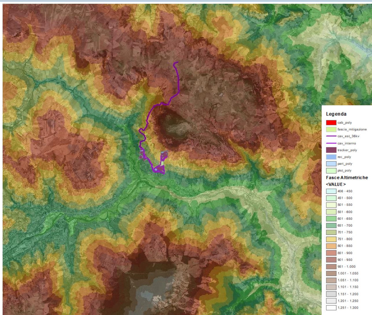
Figura 1.18. – Stralcio Carta delle fasce altimetriche.
