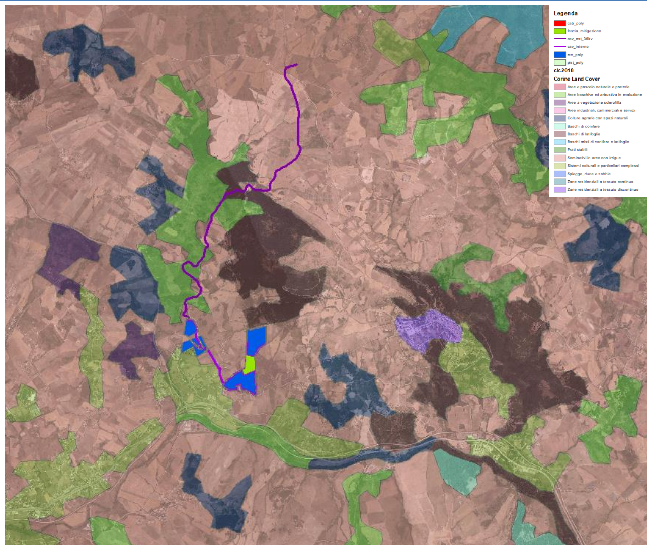
Figura 1.13. – Stralcio Carta Uso del Suolo Corine Land Cover 2018.
