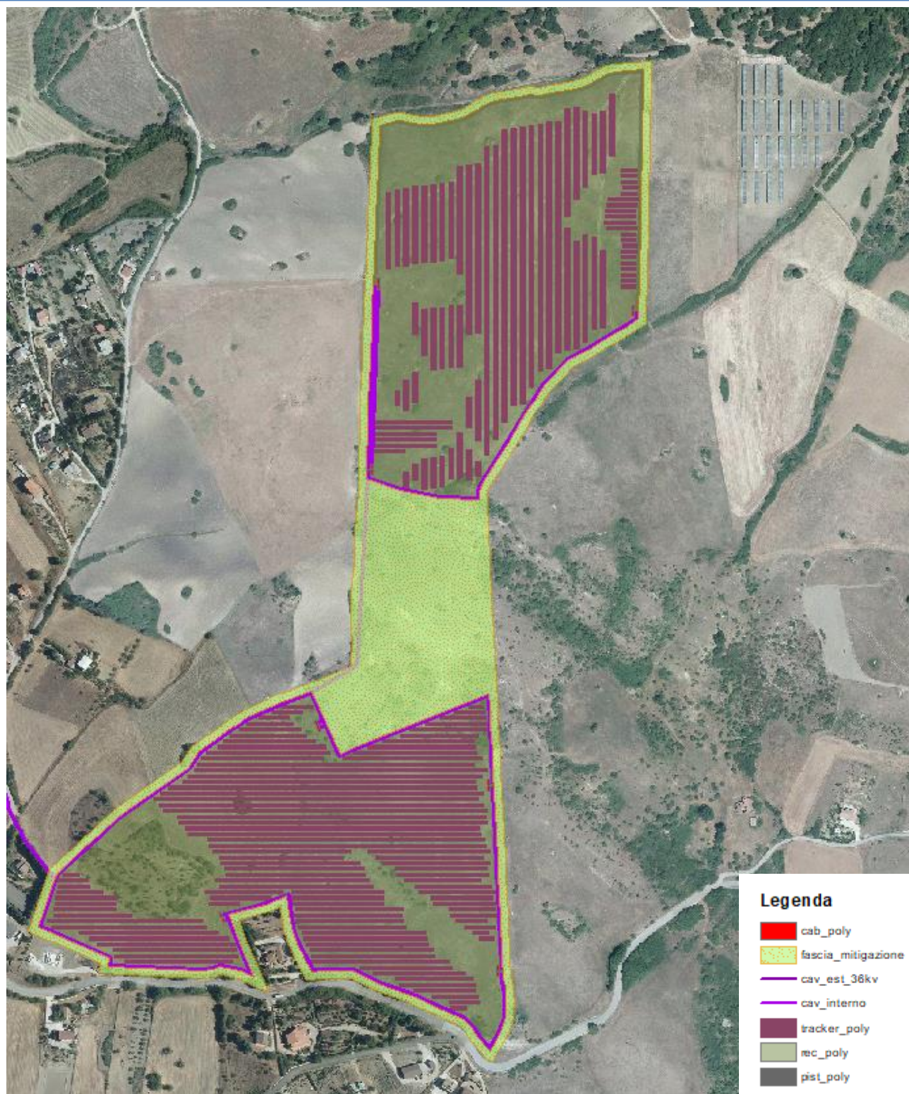
Figura 2.10a – Area di interesse dell’Impianto Agrovoltico – dettaglio.
