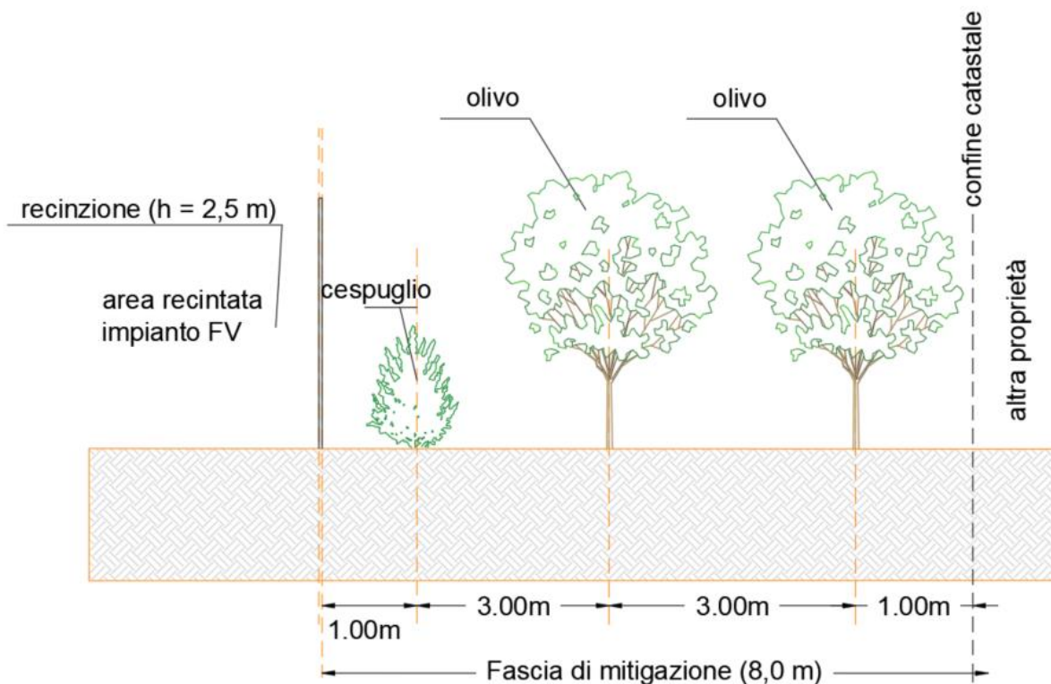
Figura 2.13. – Stralcio di sezione dell'area perimetrale dell'impianto.
