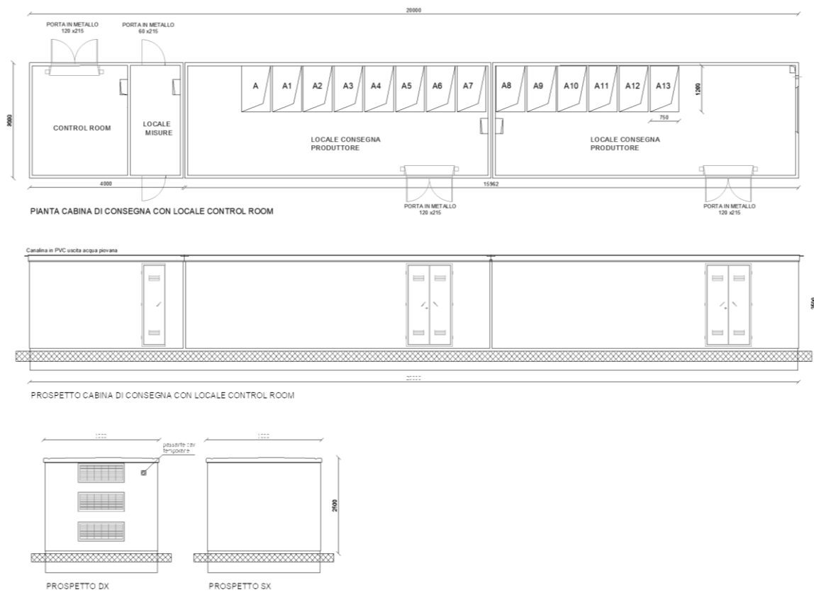
Figura 9 - Cabina di raccolta 20 m x 3 m e control room
