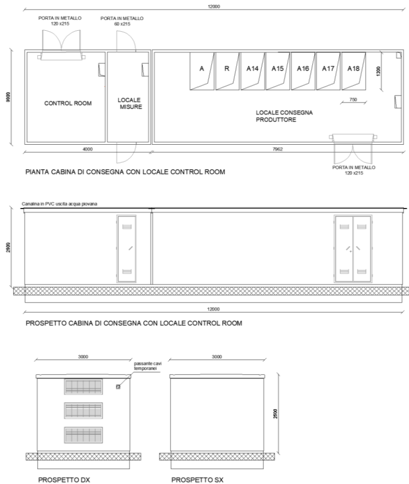
Figura 10 - Cabina di raccolta 12m x 3 m e control room
