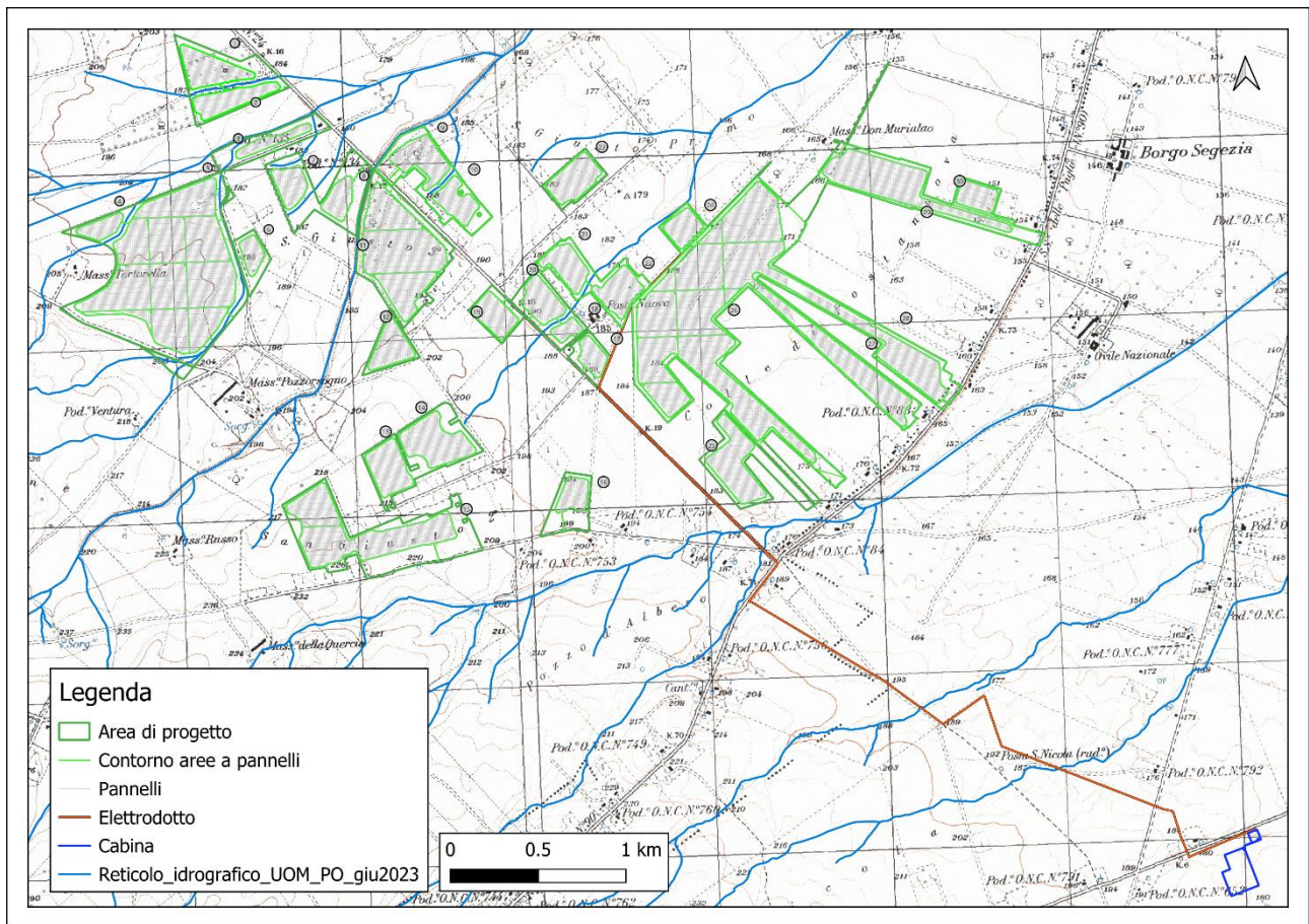
Figura 8 – Reticolo idrografico
