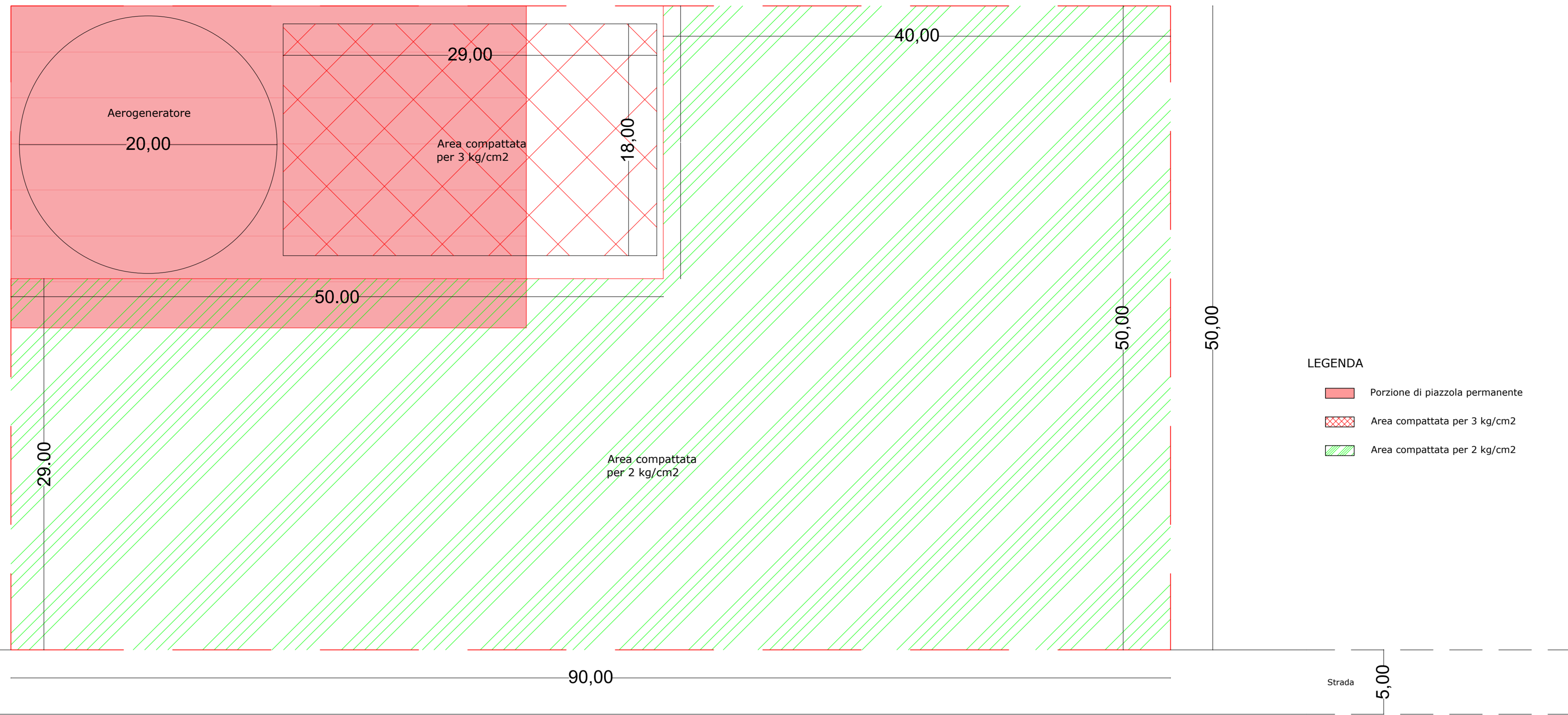
Planimetria piazzola con indicazione aree compattate
