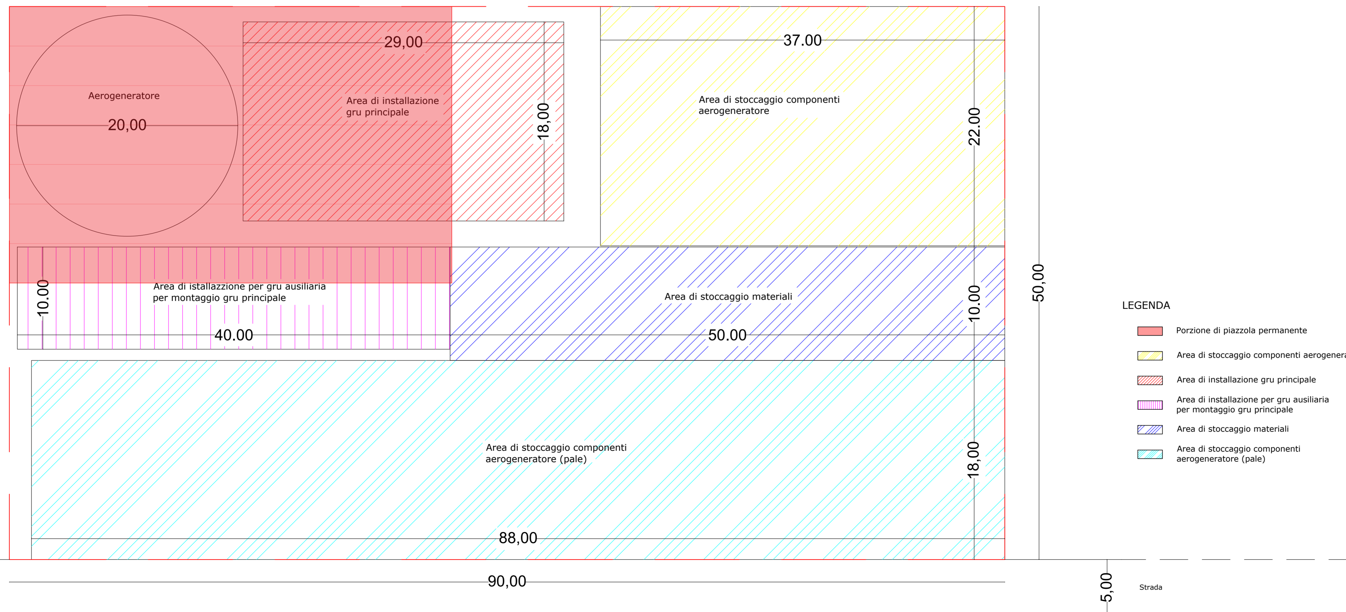
Planimetria piazzola con indicazione spazi necessari
