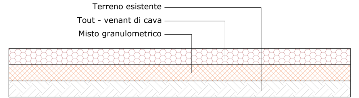
Sezione tipo finitura piazzola di montaggio
