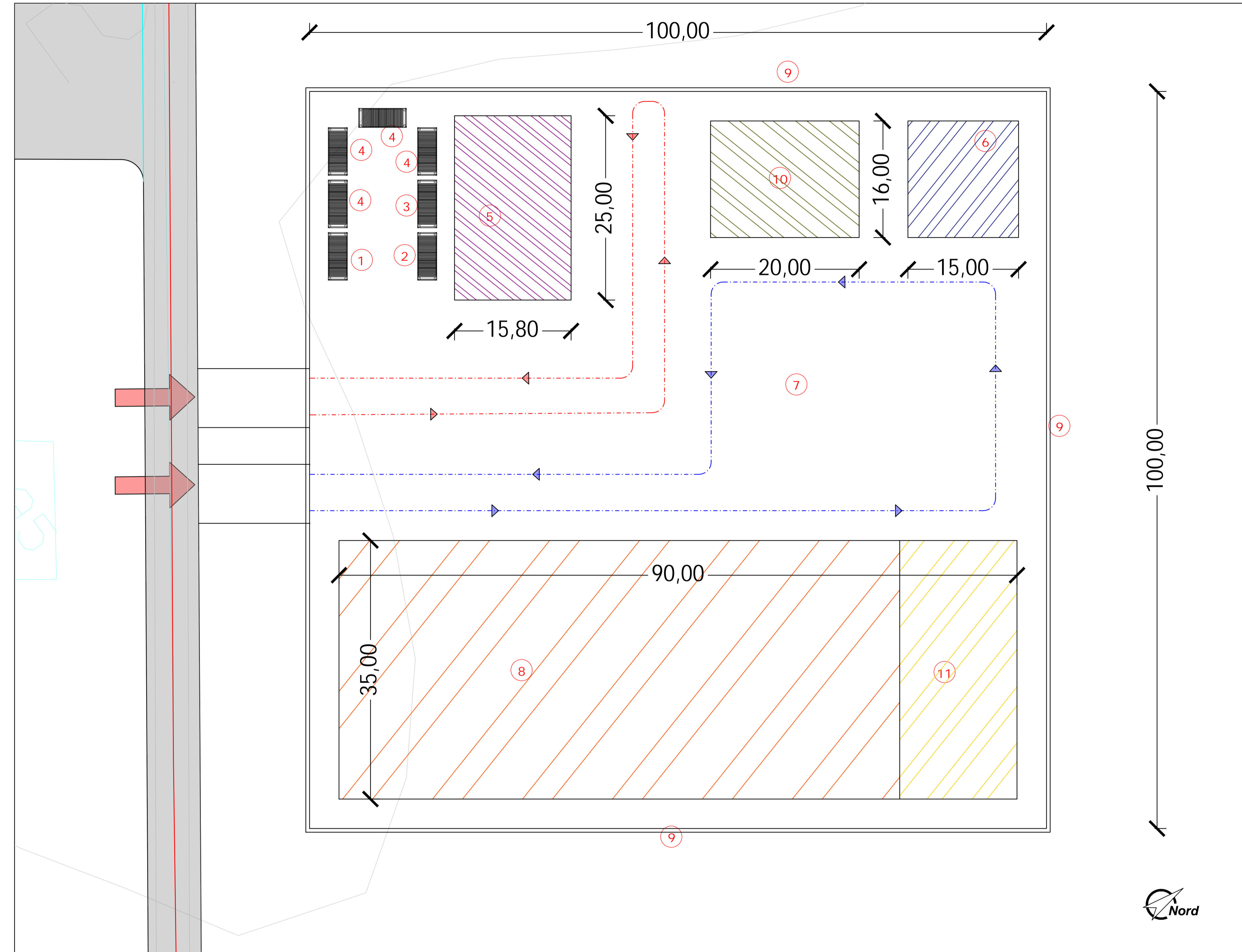
Planimetria di dettaglio
