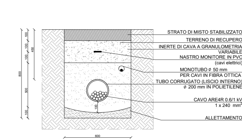
Sezione tipo "A2"
