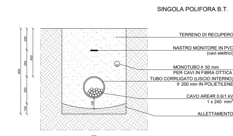
Sezione tipo "A1"
