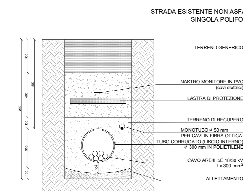
Sezione tipo "X"
