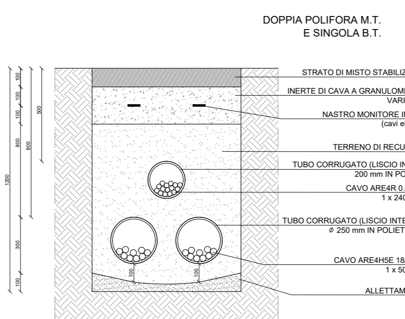
Sezione tipo "A2s"
