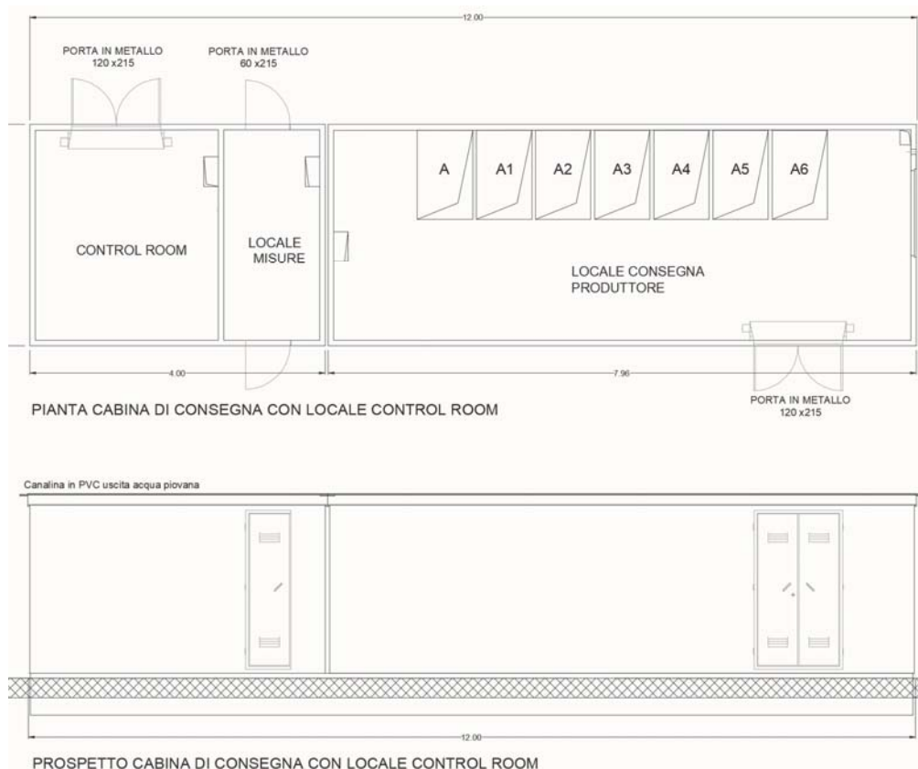
Figura 8 - Cabina di raccolta e control room
