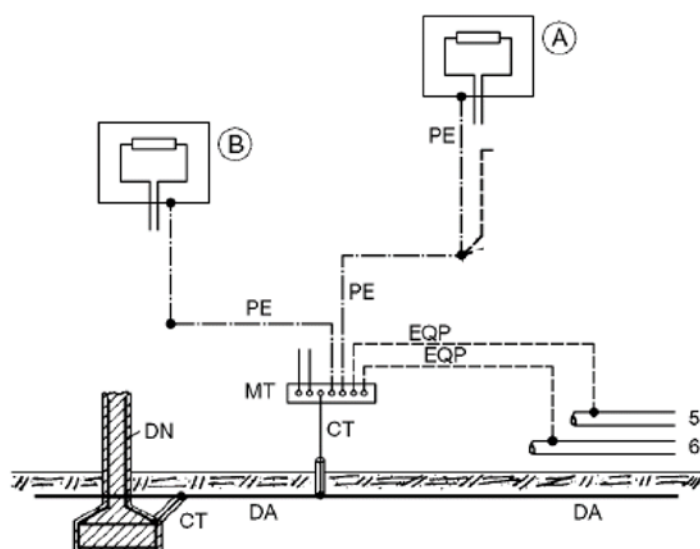
Figura 14- Esempio impianto di terra
