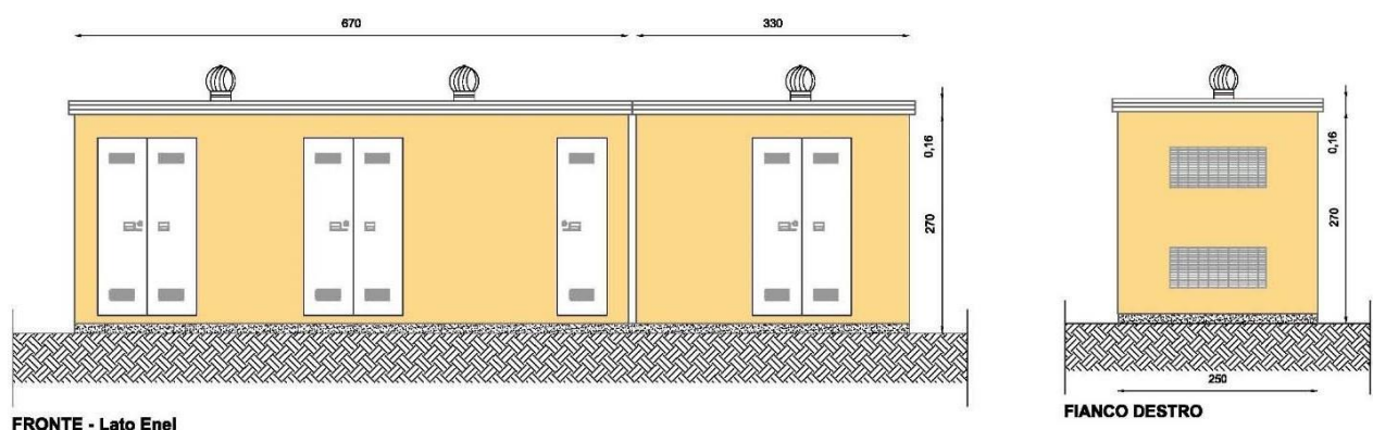
Cabina di consegna
