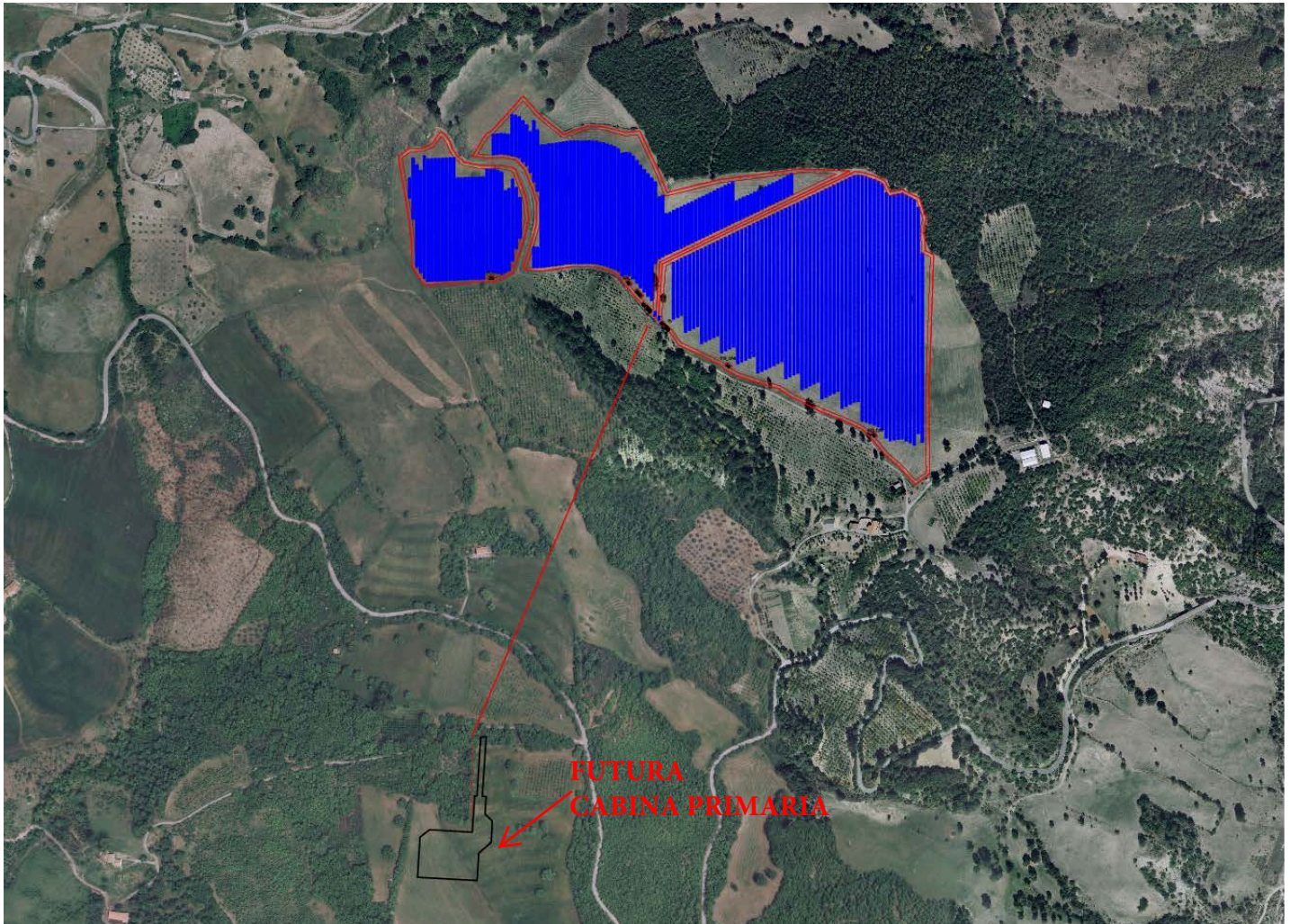
Panoramica dell'impianto e del cavidotto
