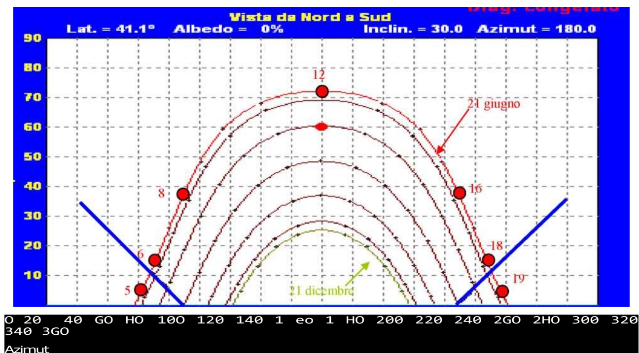
Figura 2 - Diagrammi solari della città di Bari e orari di illuminazione dei moduli FV (Elaborazione con Software Sunsim)
