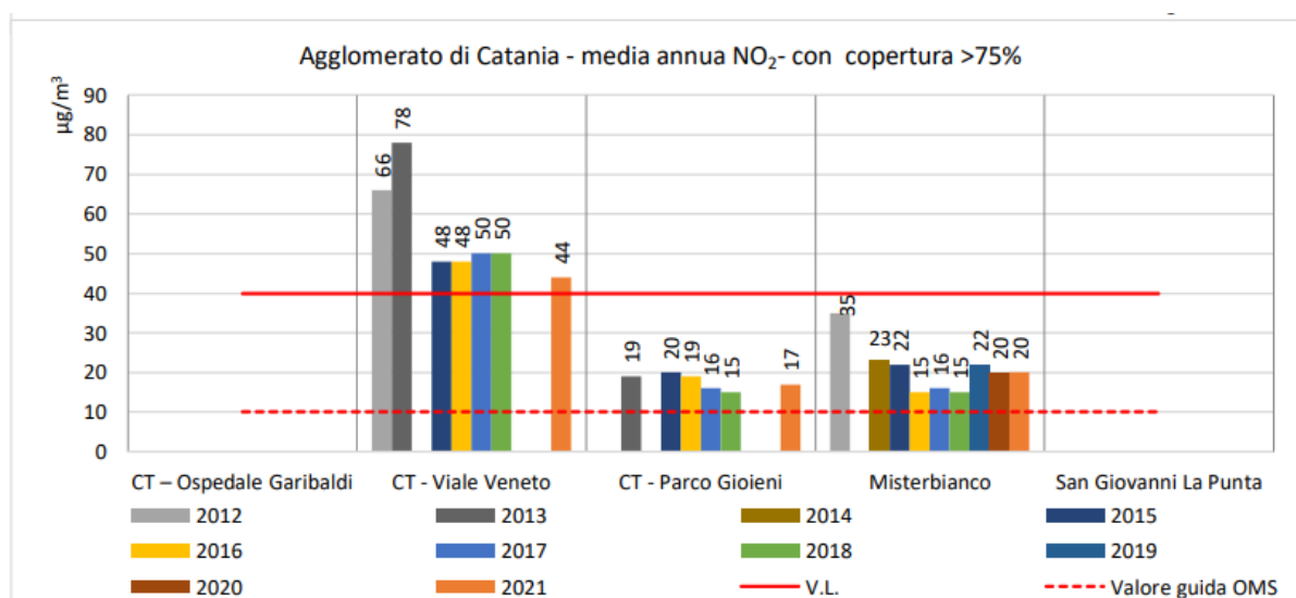
Figura 10: Media annua \text{NO}_2 - Agglomerato di Catania (Fonte: Arpa Sicilia)
