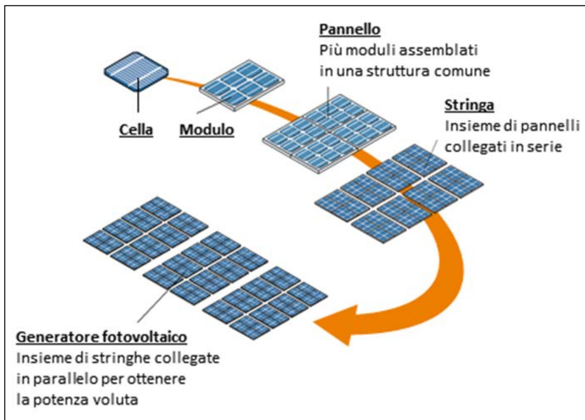
Figura 32: unità elementari del generatore fotovoltaico
