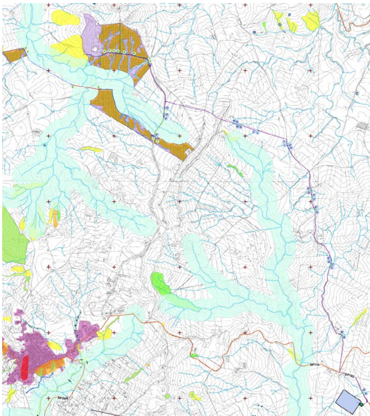
Figura 30: interferenze del parco di Raddusa (CT), da realizzare in località "Pietra Pizzata", con le infrastrutture presenti - stralcio dell'elaborato grafico "Planimetria con individuazione delle interferenze"
