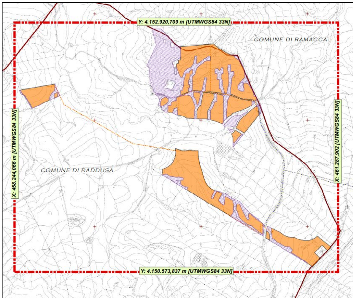
Figura 2: coordinate geografiche del perimetro racchiudente l'area di progetto fornite nel sistema di riferimento UTM WGS84 - vedasi elaborato grafico "Carta con localizzazione georeferenziata"
