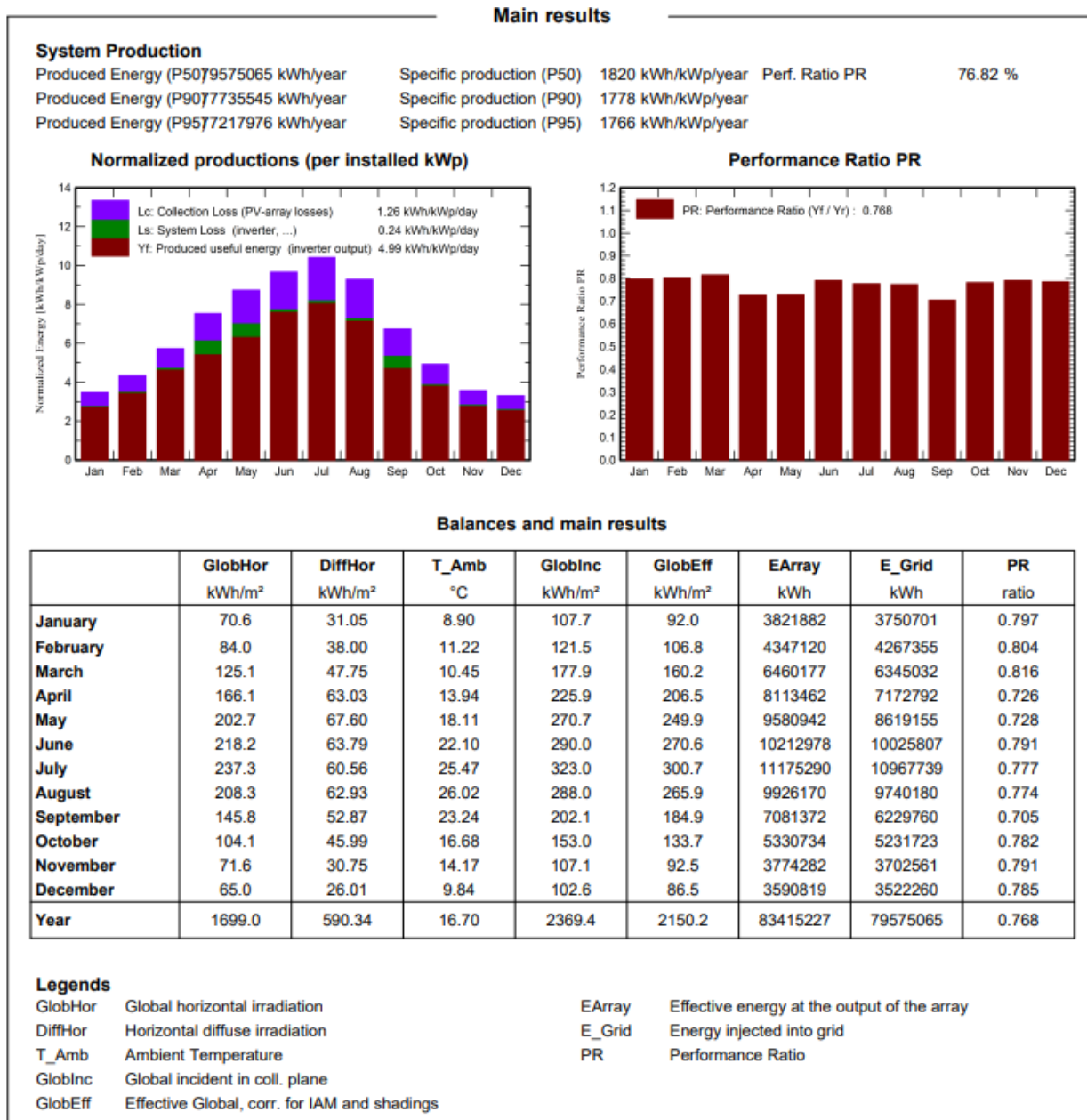
Figura 4: Risultati ottenuti con PVSyst
