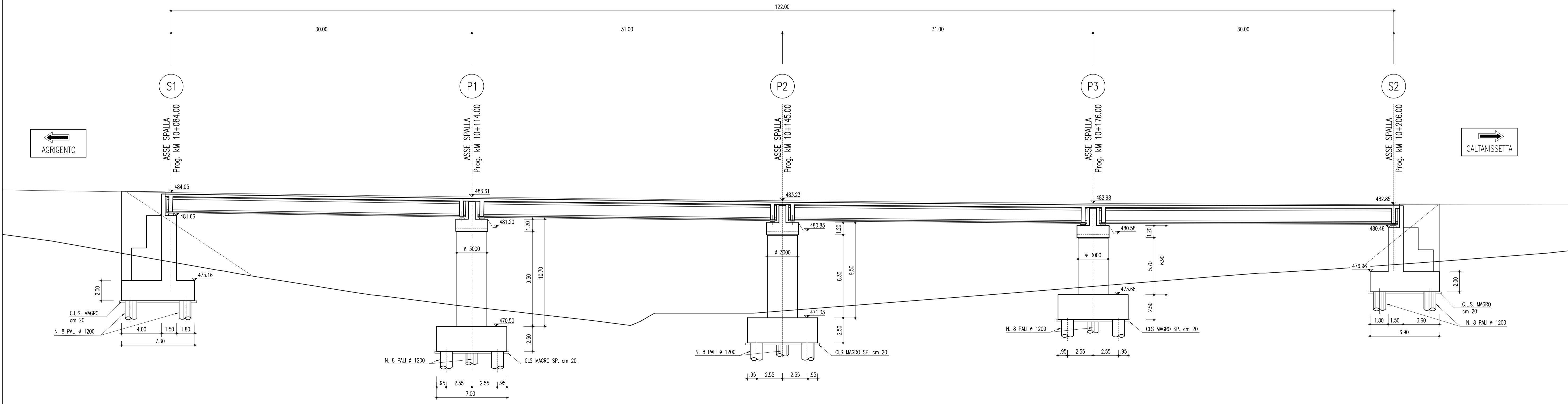
SEZIONE LONGITUDINALE PISTA DESTRA (CALTANISSETTA) SCALA 1 : 200
