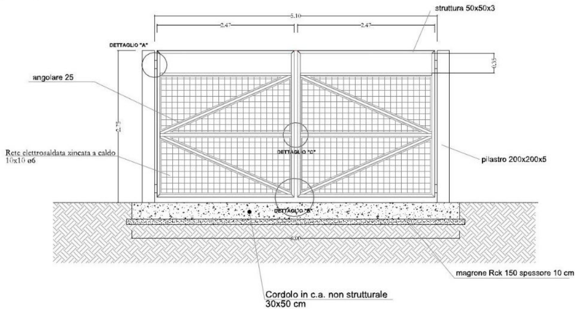
Cancello di ingresso al Parco Fotovoltaico
