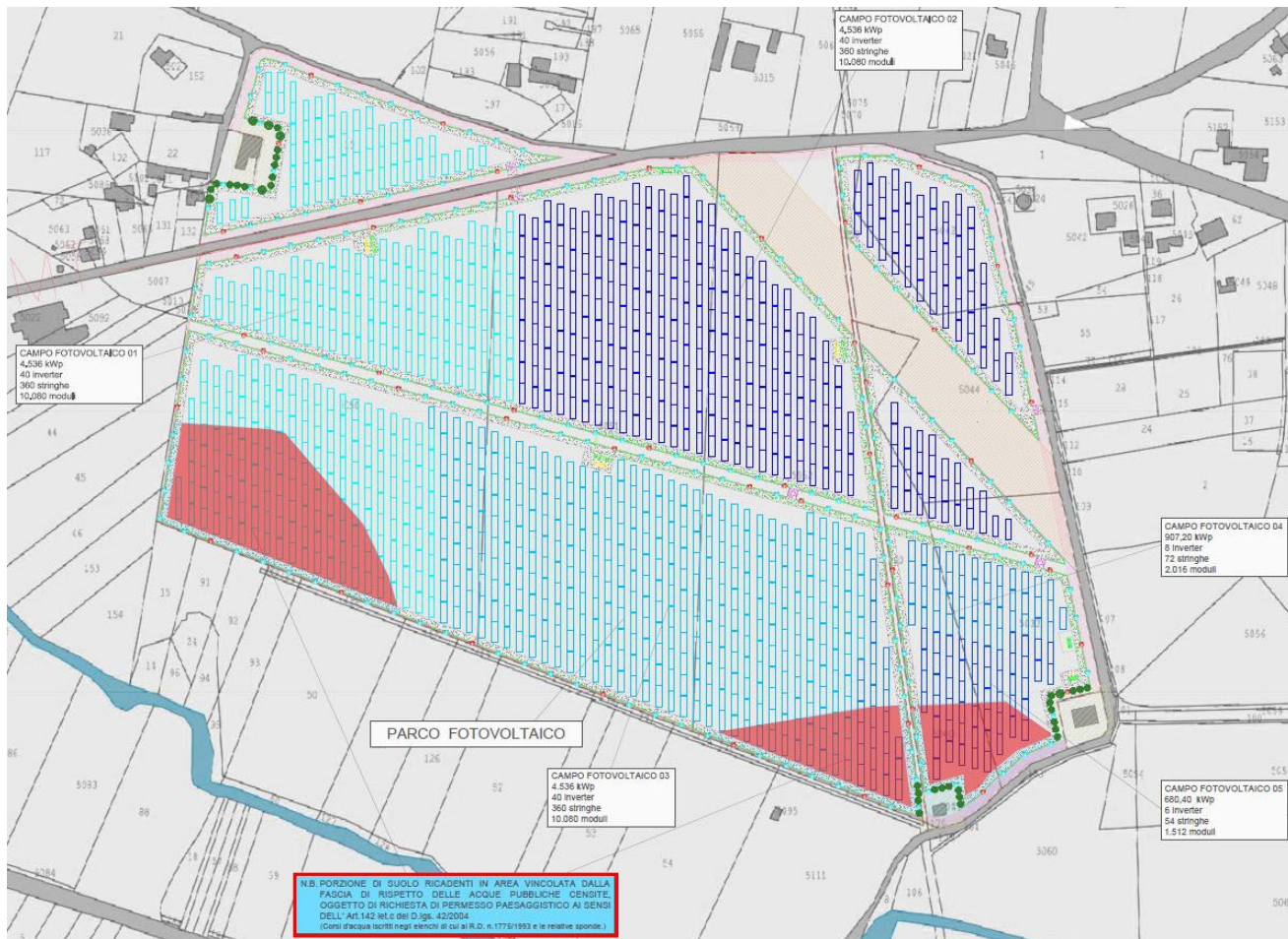
Stralcio Layout di Progetto con aree ricadenti nella fascia di rispetto del "Rio Travata"
