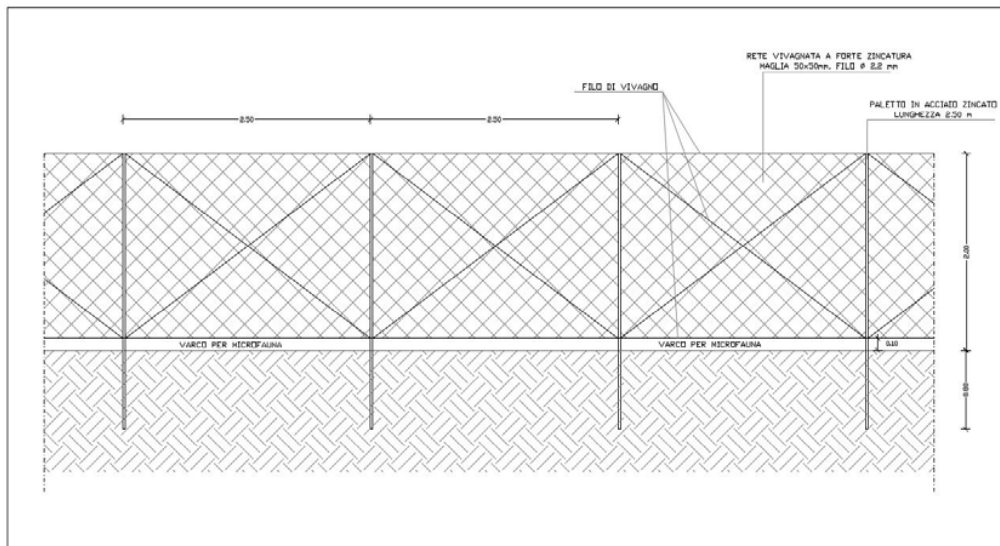
Recinzione tipo dell'Area del Parco Fotovoltaico
