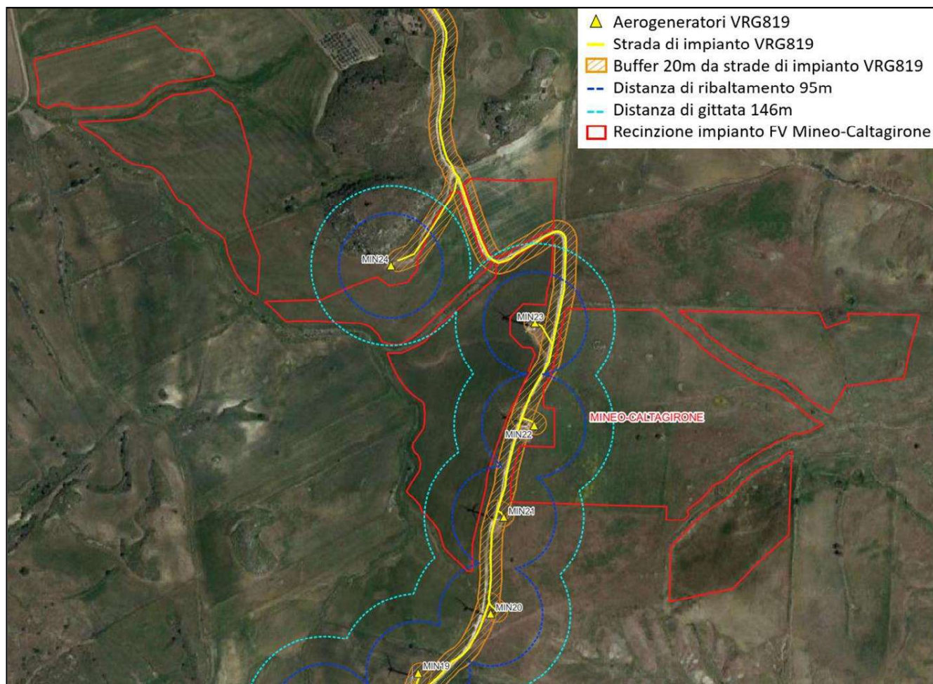
Figura 2: Sovrapposizione tra il perimetro della recinzione esterna del progetto fotovoltaico "FV Mineo-Caltagirone" e l'impianto eolico in esercizio "VRG Wind 819", con indicazione delle distanze di ribaltamento e di gittata dagli aerogeneratori esistenti e del buffer di 20 m dalle strade dell'impianto eolico esistente
