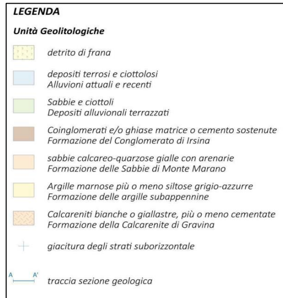
Tavola.3. – Estratto elaborato 3RGa_Carta geologica – Scala 1:10.000/5.000
