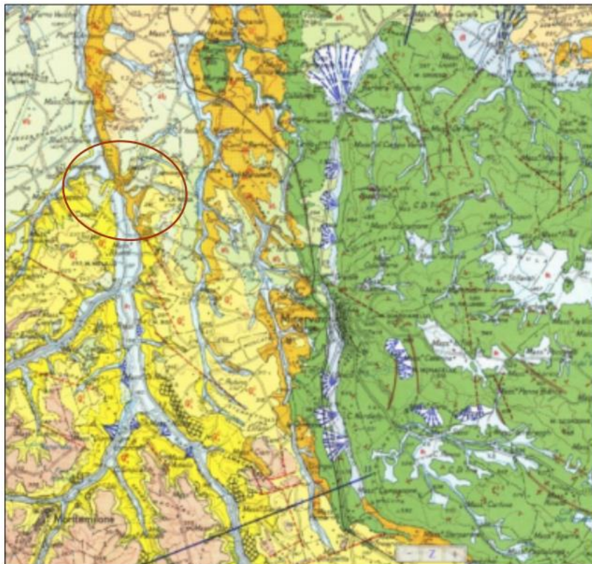
Tavola.2. - Stralcio Foglio Geologico n°176 "Barletta" in scala 1:100.000
