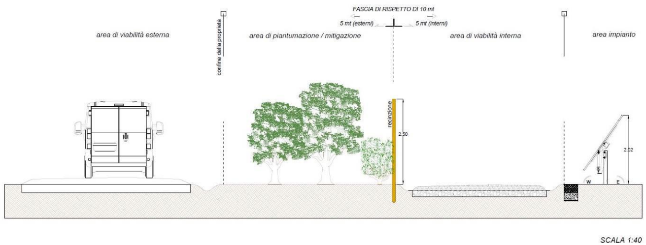
Pianta di tipica area perimetrale con piantumazione e viabilità tipica
