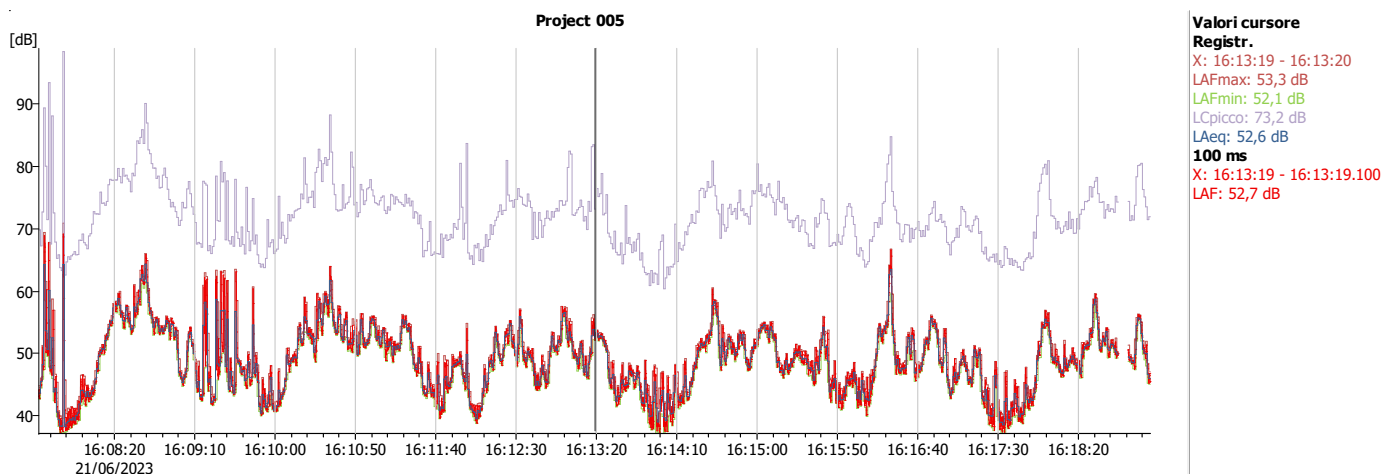
MIS 3 analisi temporale della misurazione nel punto 3
