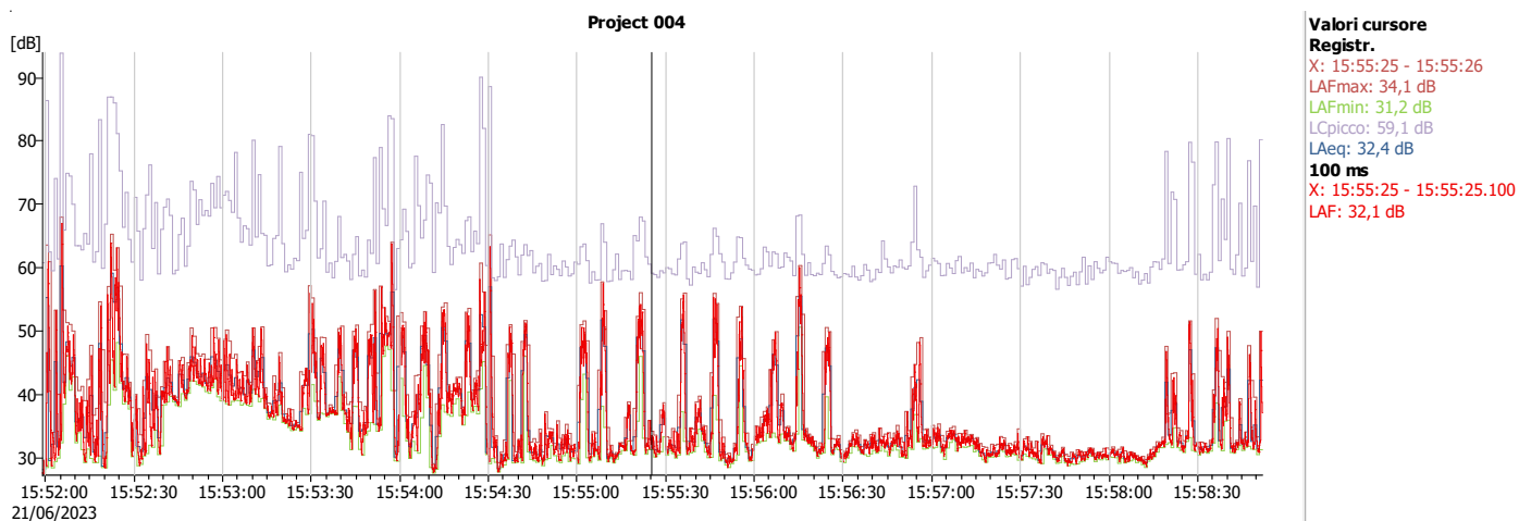
MIS 2 analisi temporale della misurazione nel punto 2
