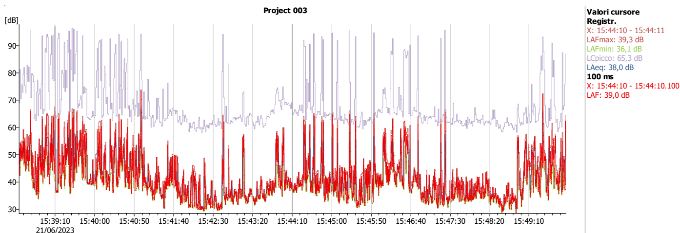
MIS 1 Grafico analisi temporale della misurazione nel punto 1
