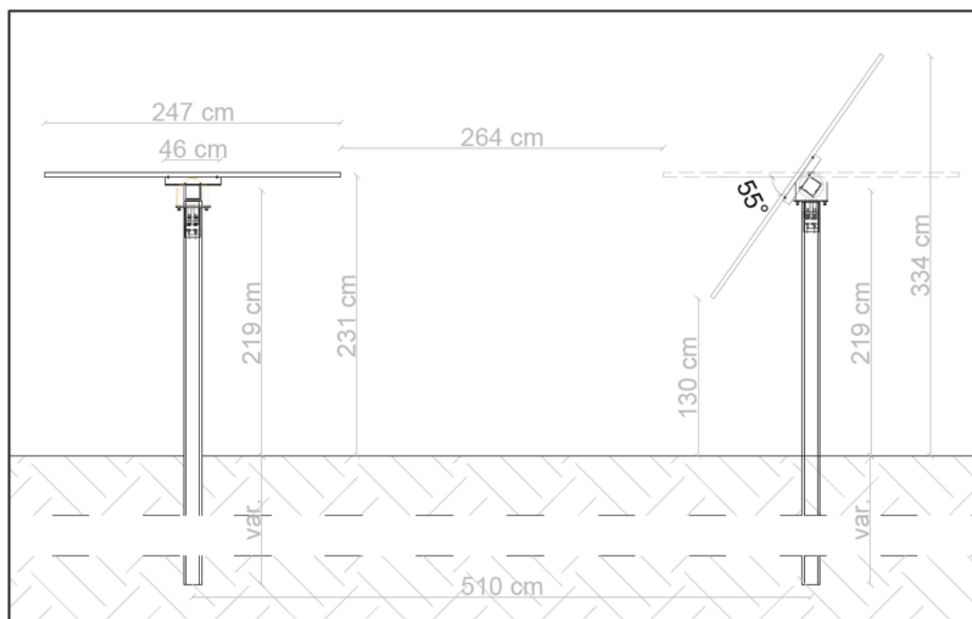
Figura 2. I Tracker porta pannelli ad asse variabile. Asse di rotazione: Nord-Sud; angolo ad inseguimento su singolo asse (tracker): da +55^\circ a -55^\circ .
