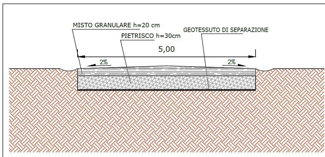
Figura 3. La sezione tipo di realizzazione della viabilità interna all'impiantistica fotovoltaica.
