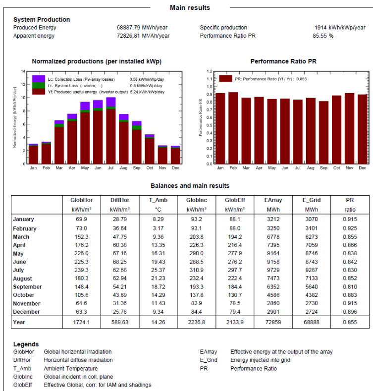
FIGURA 8: PRODUCIBILITA' ELETTRICA DELL'IMPIANTO AGRIVOLTAICO VALUTATA TRAMITE PVSYS
