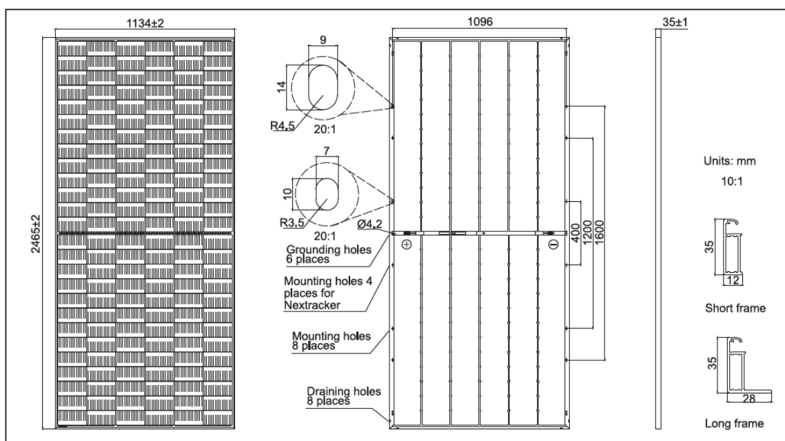
FIGURA 11: PANNELLO FV PARI A 625 WP CON DIMENSIONI 2465 X 1134 X 35 MM
