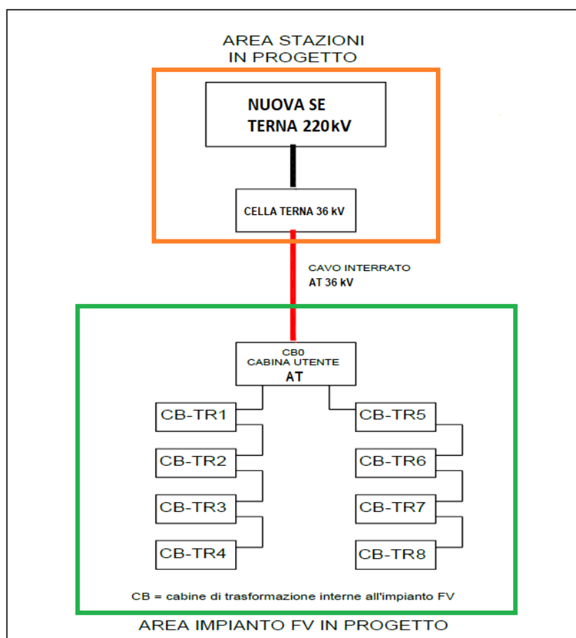
FIGURA 10: SCHEMA A BLOCCHI IMPIANTO
