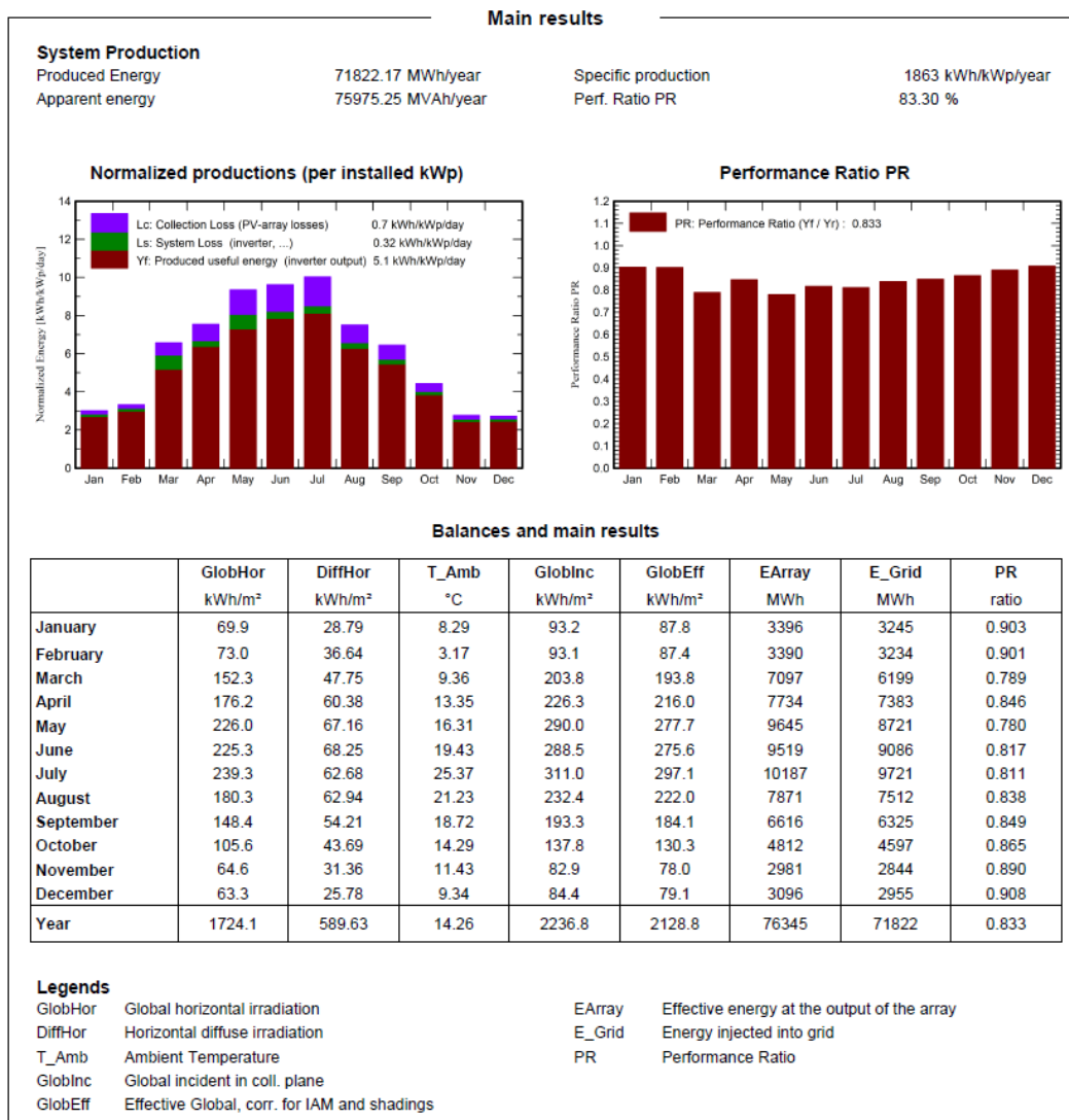
FIGURA 9: PRODUCIBILITA' ELETTRICA DELL'IMPIANTO FOTOVOLTAICO STANDARD VALUTATA TRAMITE PVSYS
