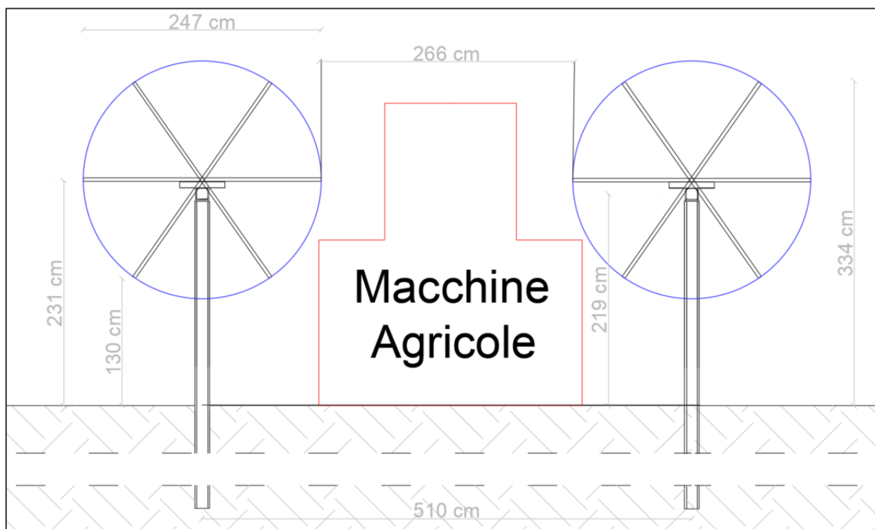
FIGURA 7: CONFIGURAZIONE STRUTTURE AD INSEGUIMENTO IMPIANTO AGRIVOLTAICO
