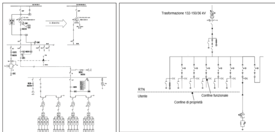
FIGURA 12: SCHEMA DI CONNESSIONE GENERALE CON PIÙ UTENTI ATTIVI (ESTRATTO DA ALLEGATO A.68 DEL 19 MAGGIO 2022)
