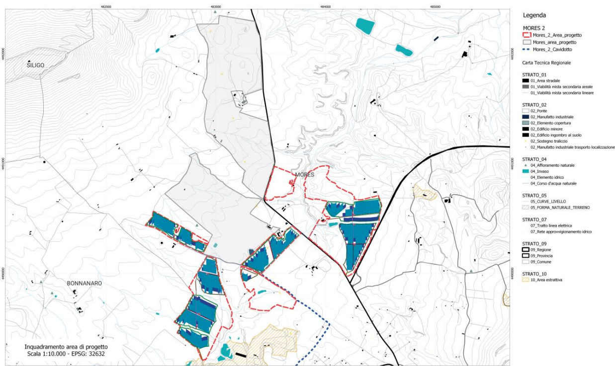
FIGURA 1: INQUADRAMENTO SU CTR IN SCALA 1:10000
