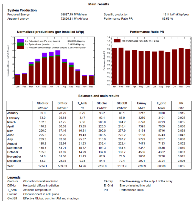
FIGURA 6: PRODUCIBILITA' ELETTRICA DELL'IMPIANTO AGRIVOLTAICO VALUTATA TRAMITE PVSYS
