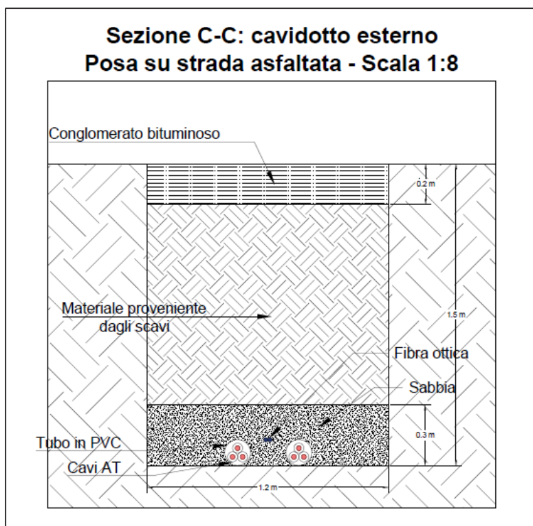
FIGURA 11: ESEMPI DI POSA CAVIDOTTO AT CONSEGNA ENERGIA
