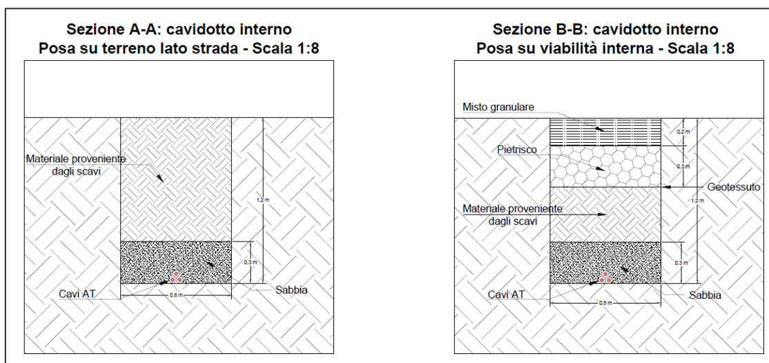
FIGURA 10: ESEMPIO POSA CAVI AT PER SERVIZI INTERNI
