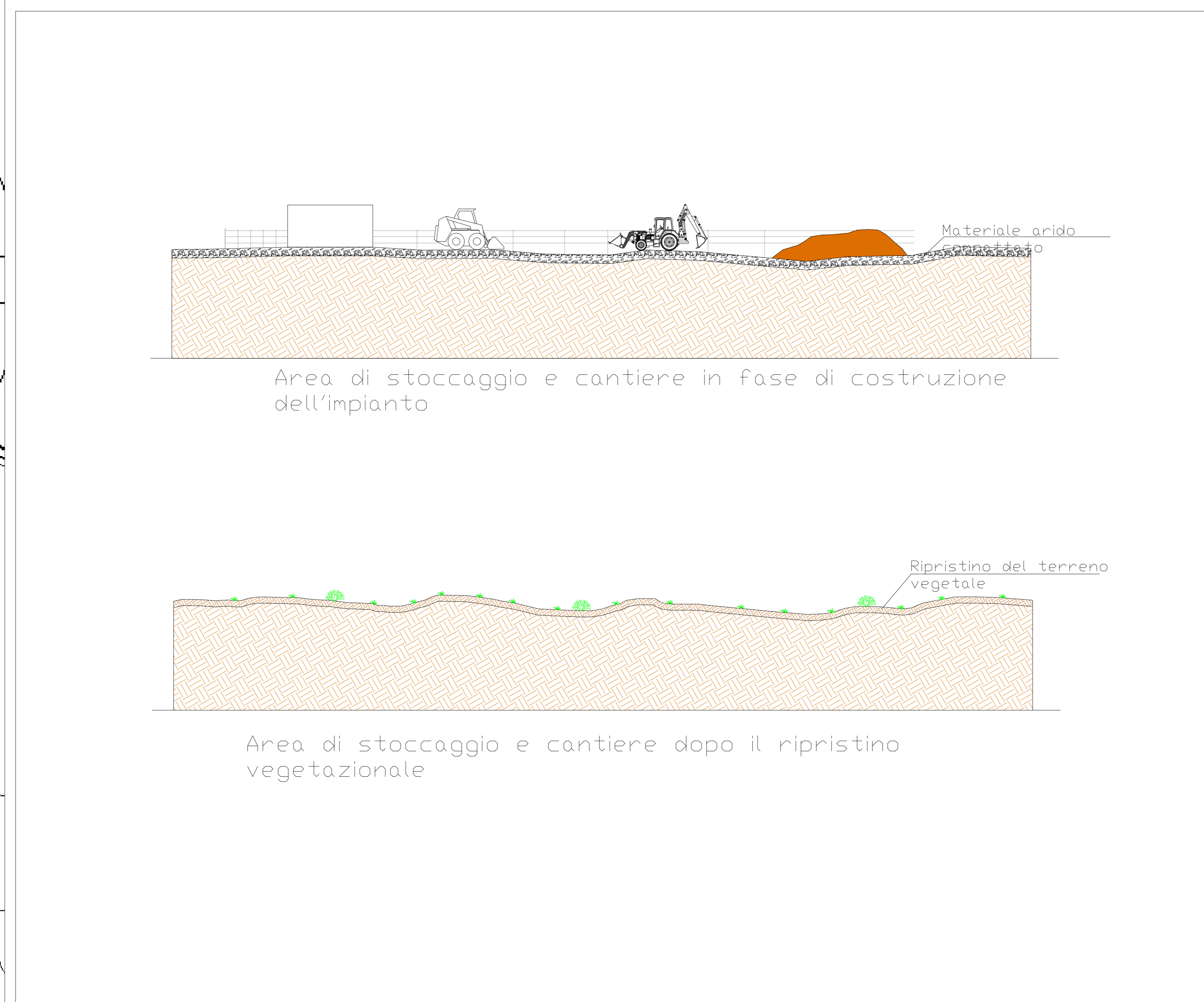
SEZIONE DELL'AREA DI STOCCAGGIO E CANTIERE (SITE CAMP)
