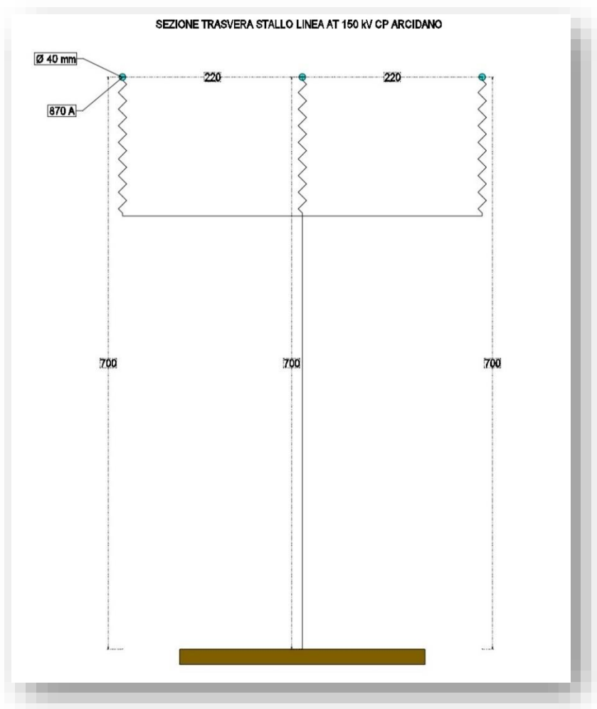
Figura 1 - schematico sezione trasversale sbarre AT stazione utente
