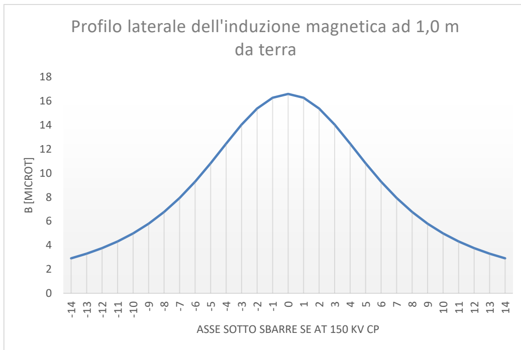
Figura 2 - Profilo CM interno all'area di stazione produttore
