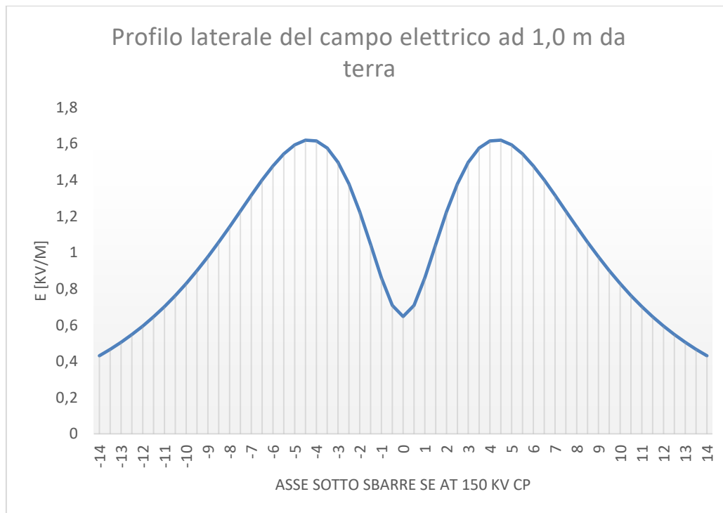
Figura 3 - profilo CE interno all'area di stazione utente
