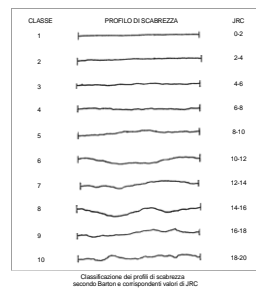
Figura 9.1 – Profili di scabrosità dei giunti
