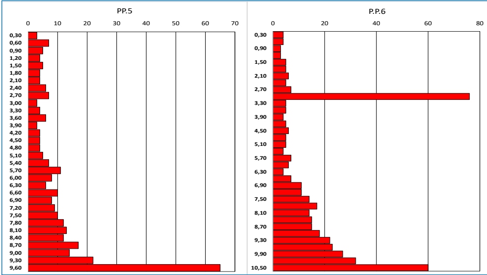
Figura 4.3 – Prove DPSH - PP.5 e PP.6
