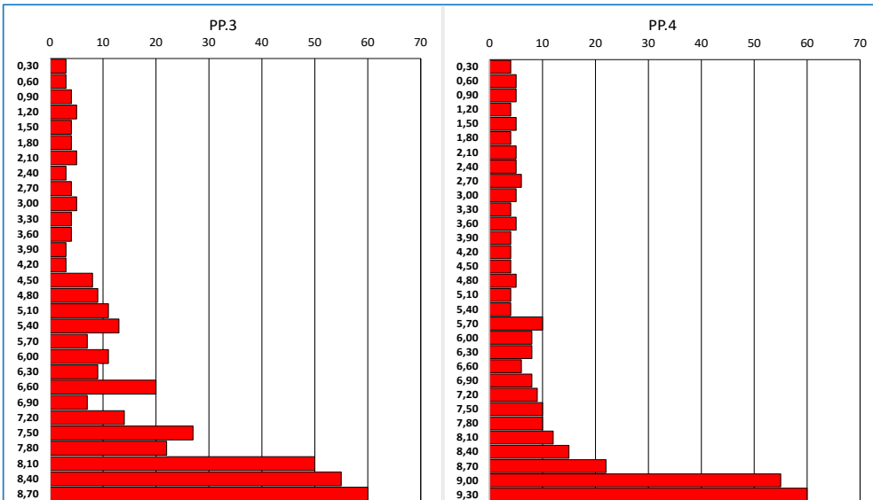
Figura 4.2 – Prove DPSH - PP.3 e PP.4
