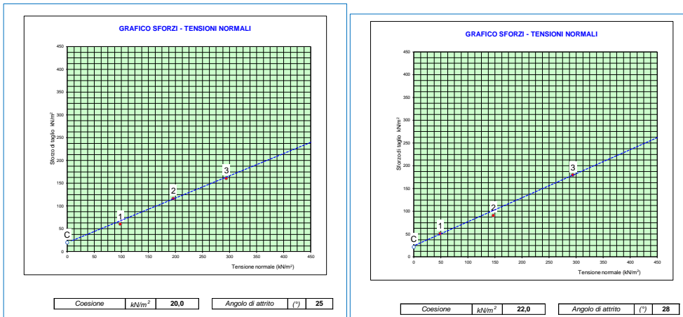
Figura 10.1 – Prova di TD (sx) - Sondaggio S.1 Campione CR1 (m11,20-11,70) e Prova di TD (dx) - Sondaggio S.3 Campione C11 (m2,00-2,50)
