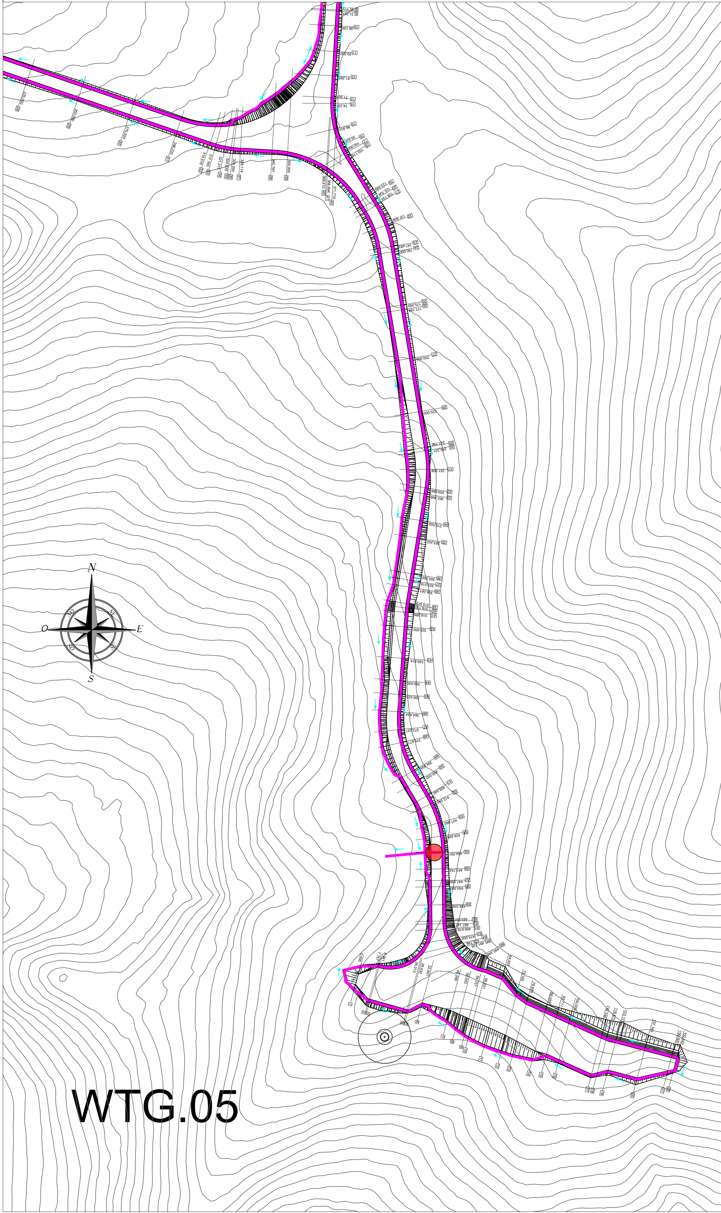
PLANIMETRIA DI DRENAGGIO WGT05 _SCALA 1:1.000
