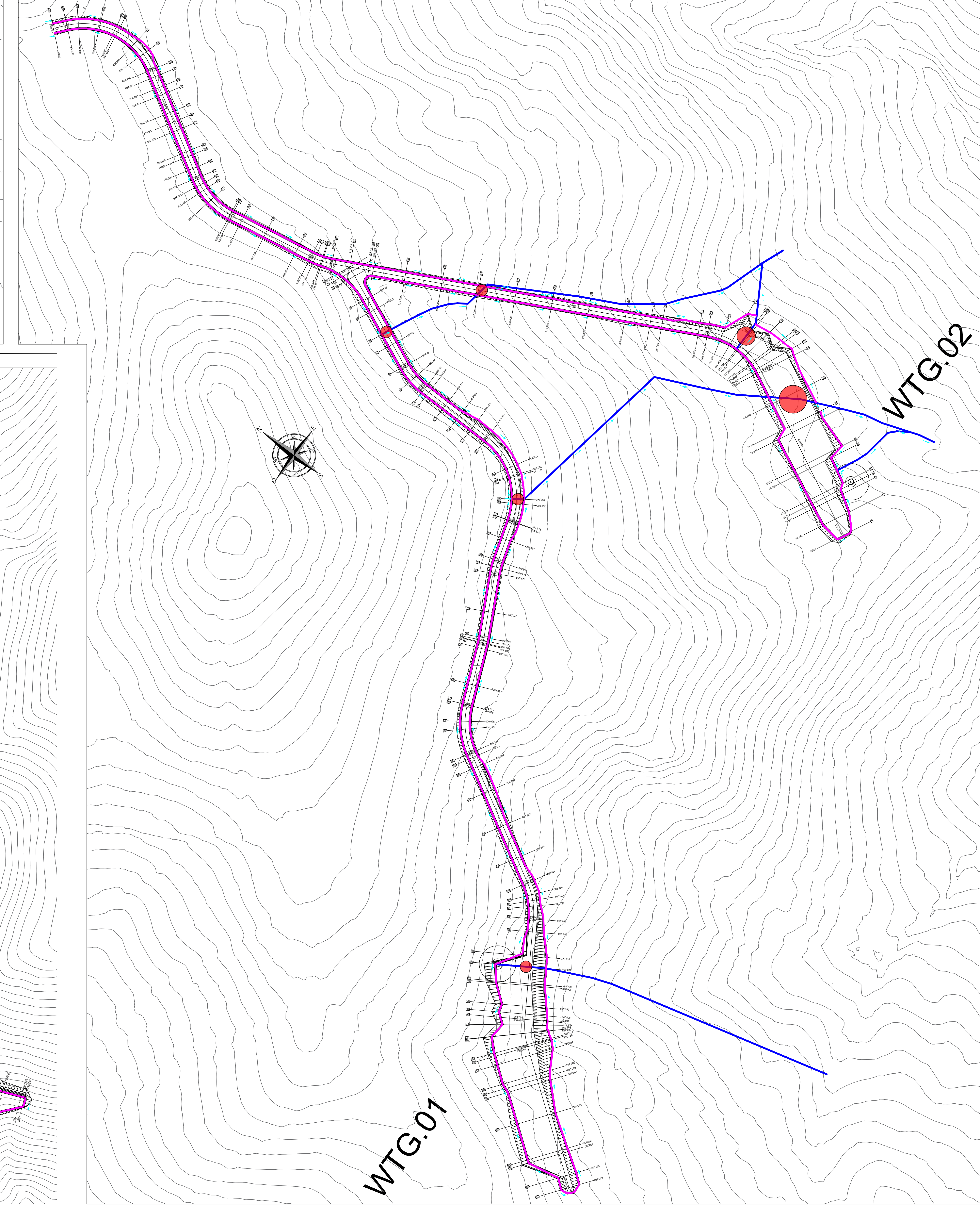
PLANIMETRIA DI DRENAGGIO WGT02 _SCALA 1:1.000
