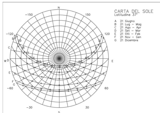
Fig. 2 - traiettorie solari - Carta del Sole Lat. 37
