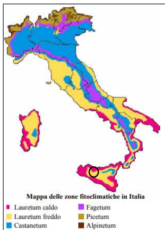
Figura 6 .5 Mappa Zone Fitoclimatiche
