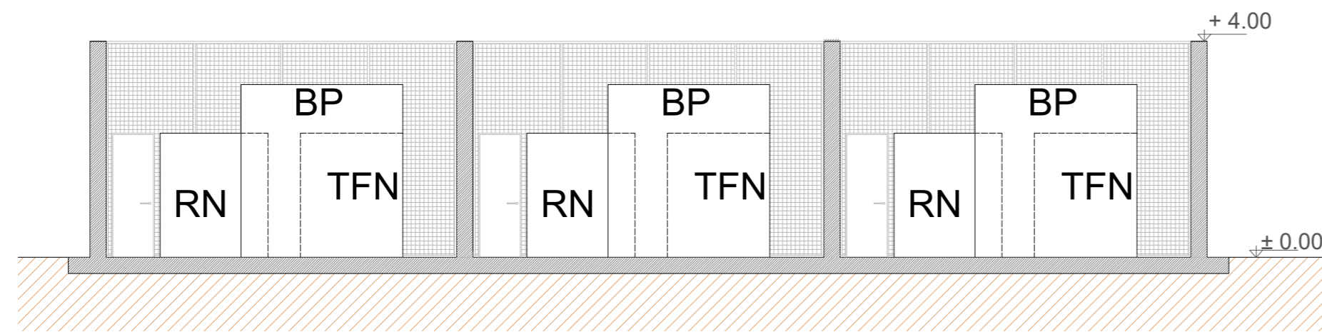
Sezione A-A
