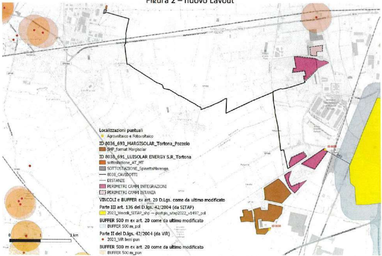
Figura 2 – nuovo Layout
