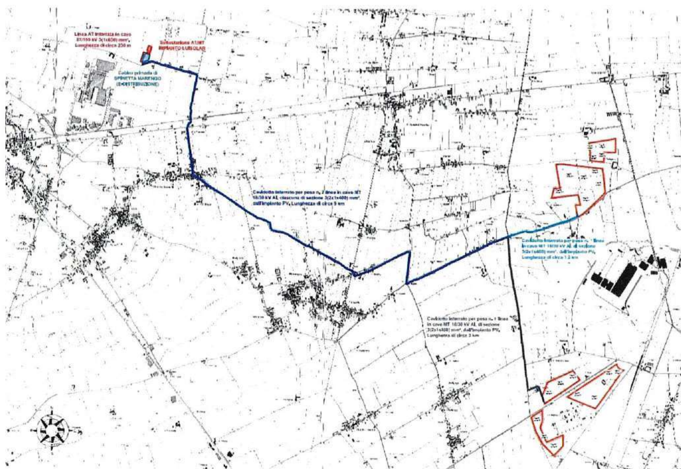
Figura 1 – Layout depositato
