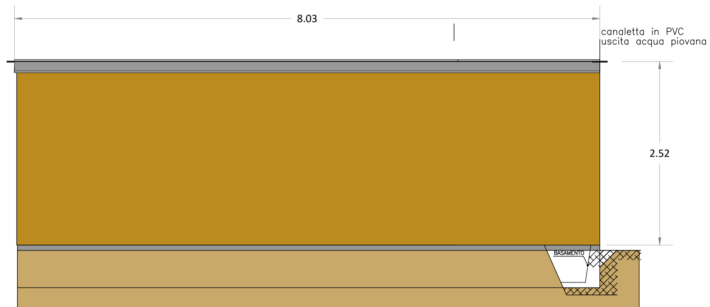
VISTA TERGALE
