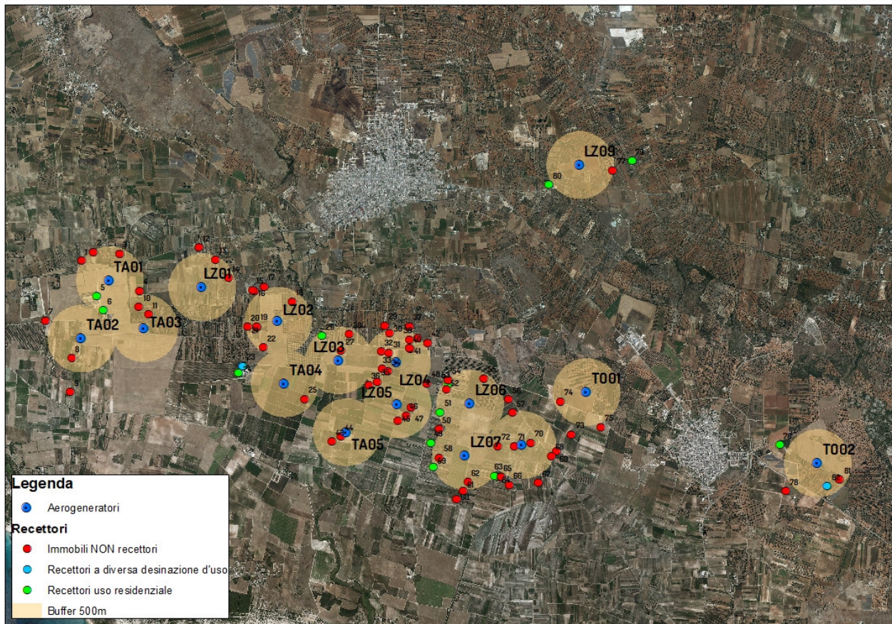
Figura 1: Postazioni di misura nei pressi dei ricettori
