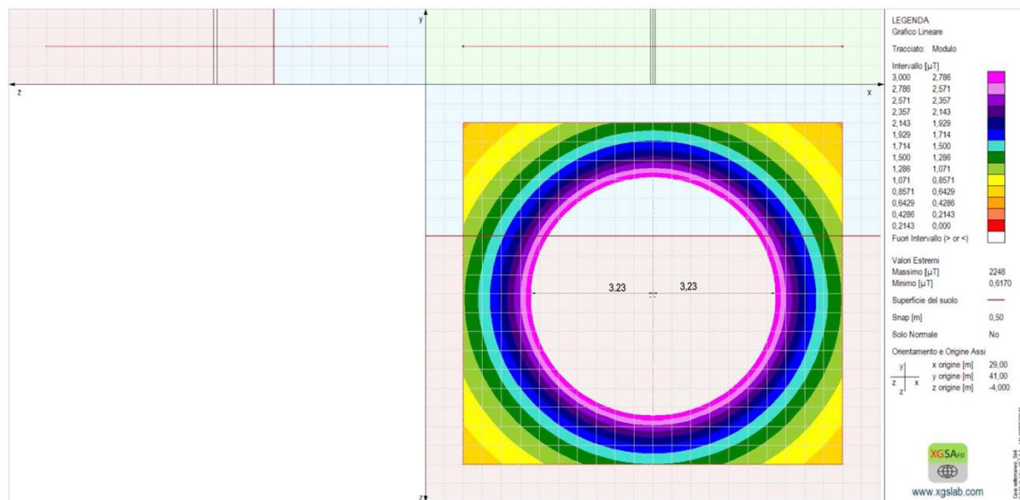
Calcolo Indizione Magnetica sulla sezione del cavo AT da 1600 mm 2
