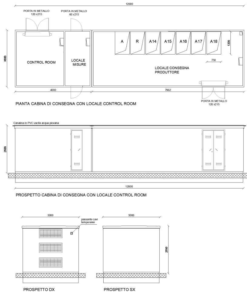
Figura 9 - Cabina di raccolta RT1 e control room
