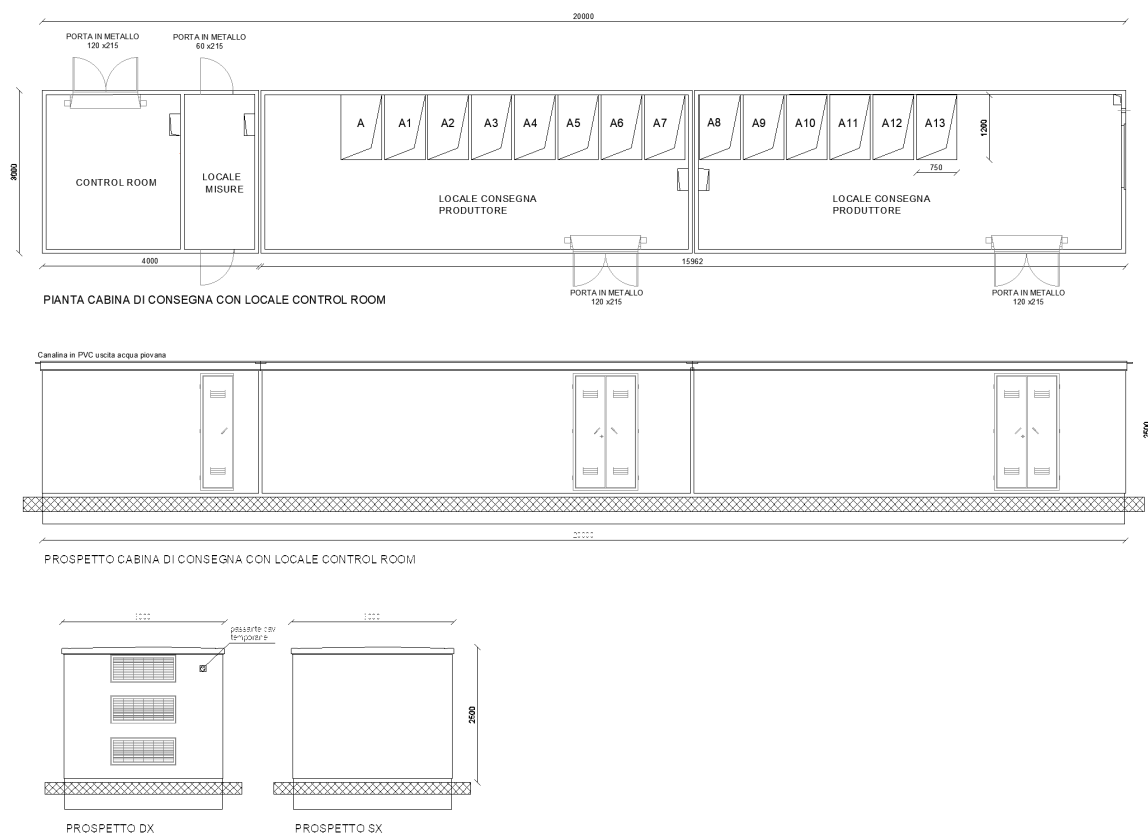
Figura 8 - Cabina di raccolta R1 e control room
