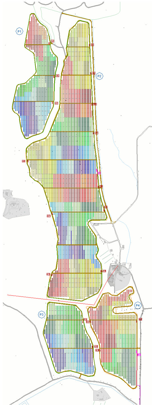
Figura 5- Particolare schema di suddivisione stringhe impianto
