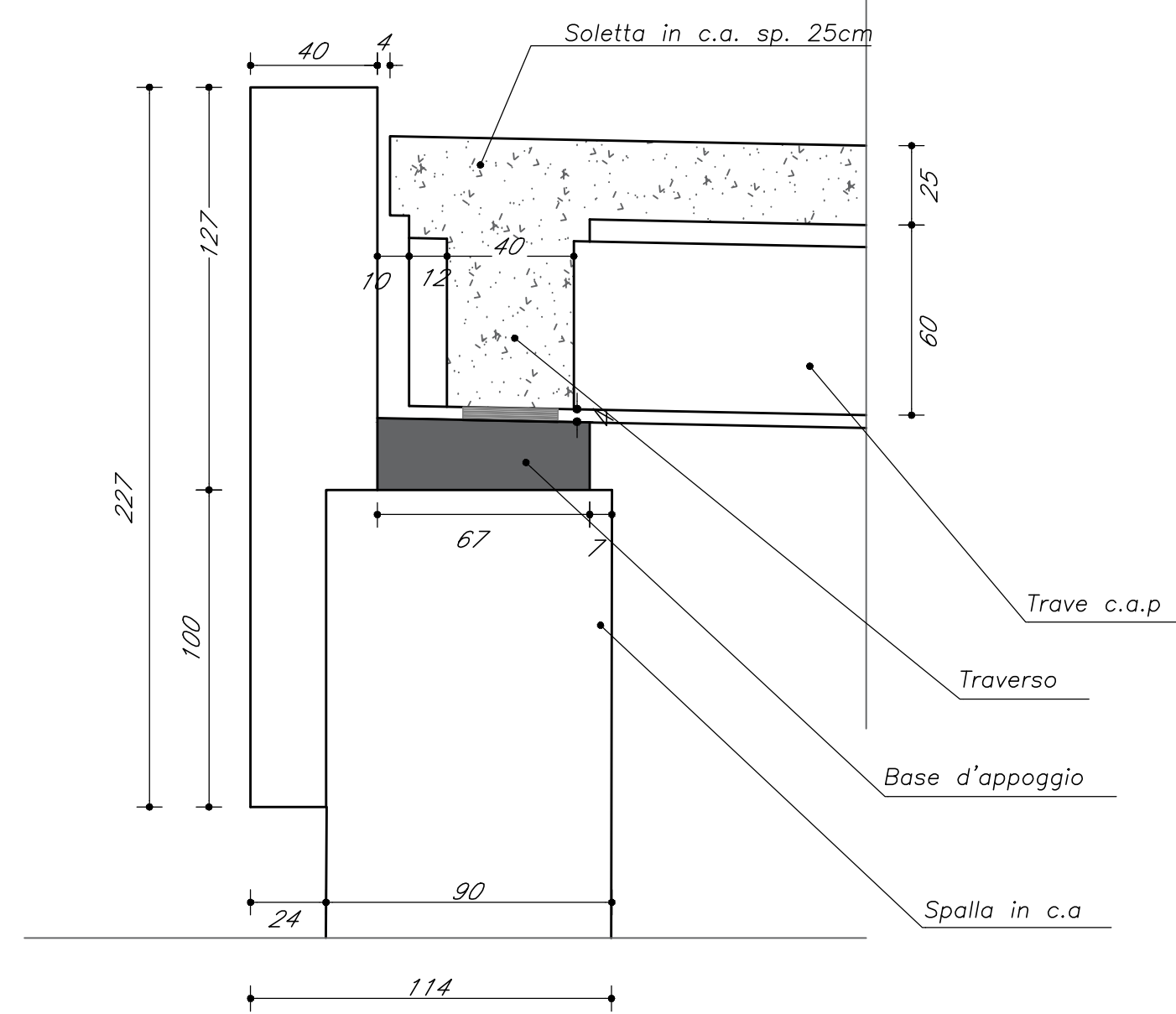
APPOGGIO TRAVE SPALLA SCALA 1:20
