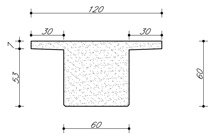
DETTAGLIO TRAVE SCALA 1:20
