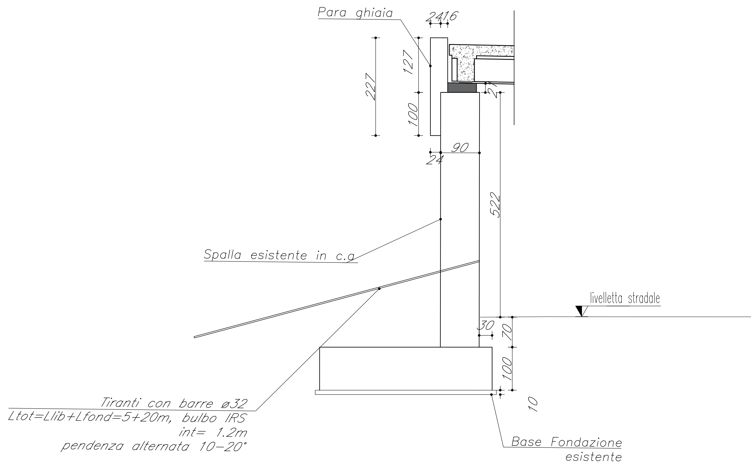
SEZIONE SPALLA ESISTNTE SCALA 1:50
